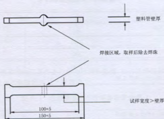
图 D.2 拉伸实验试样尺寸图
