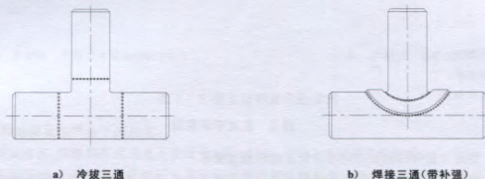
图 4 三通示意图
