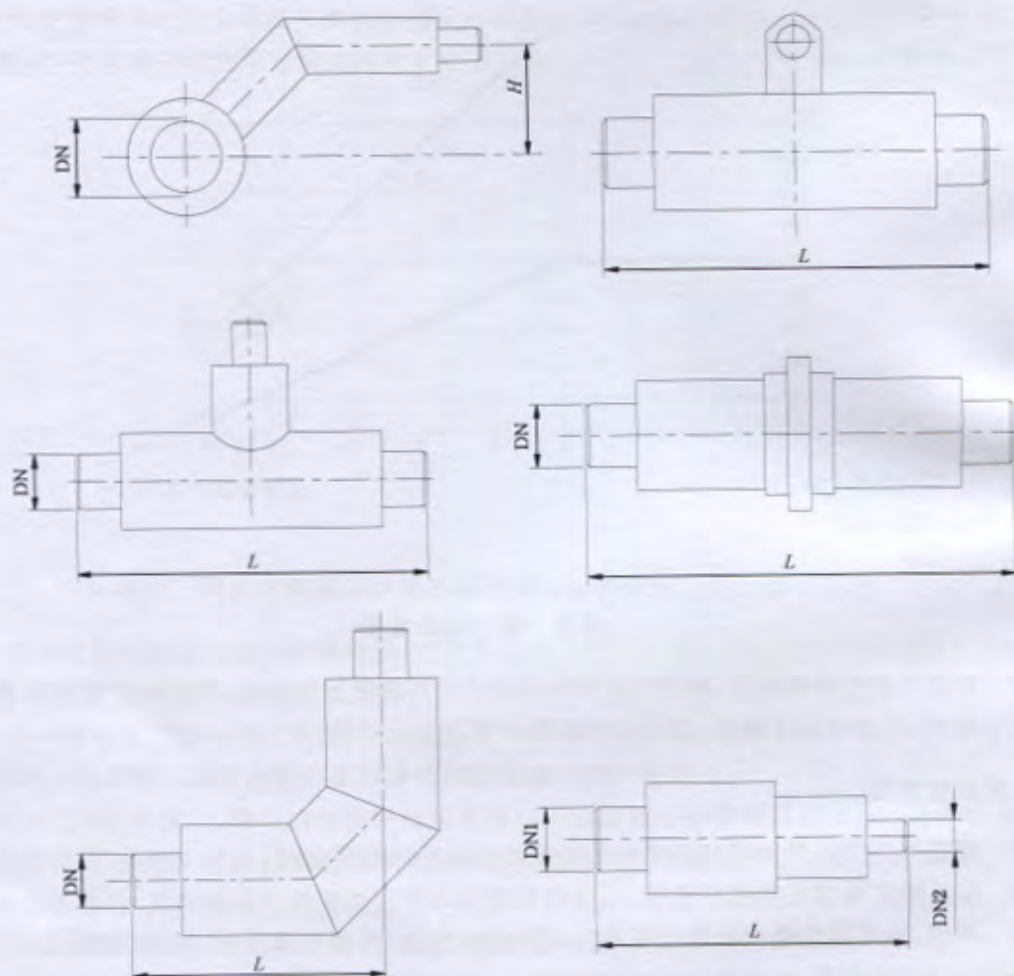
图 10 保温管件主要尺寸允许偏差示意图
