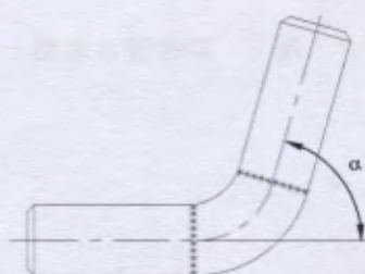
图 3 弯曲角度示意图
