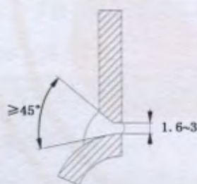
a) X 剖面 直角直管
