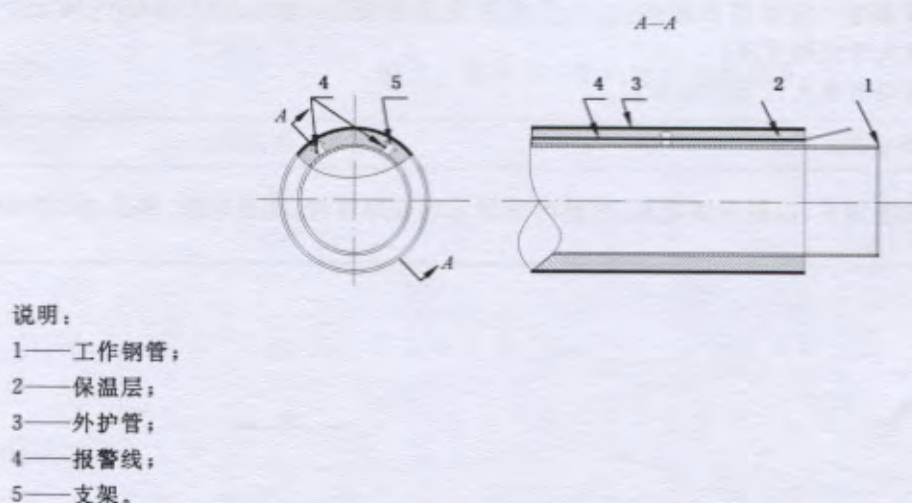
图 1 产品结构图
