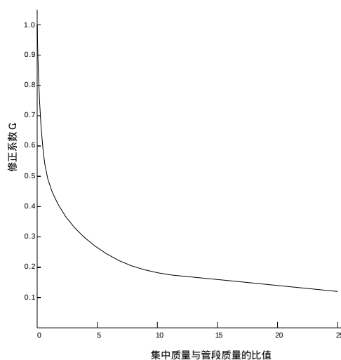
图 B.1 管道特征跨距间补偿集中质量影响的修正系数 C_1
