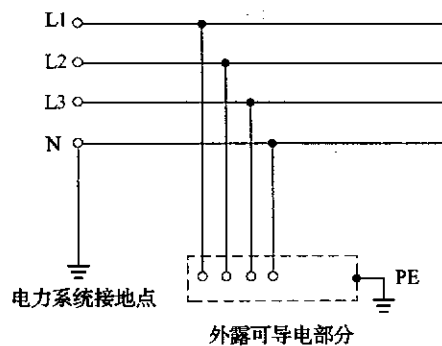
图 8 TT 系统
