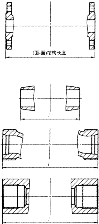
图 1 直通式阀门结构长度
