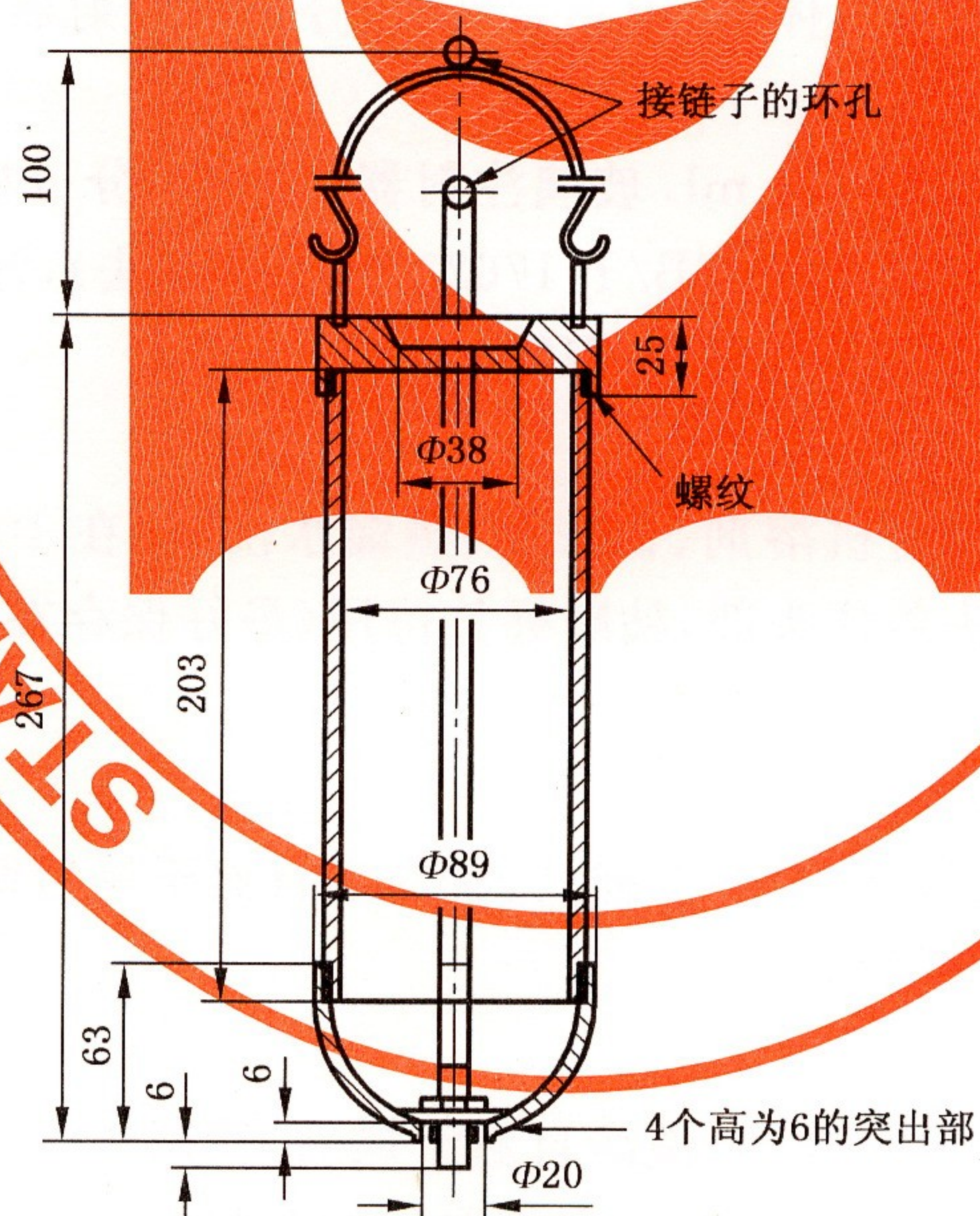
图 2 取样勺
