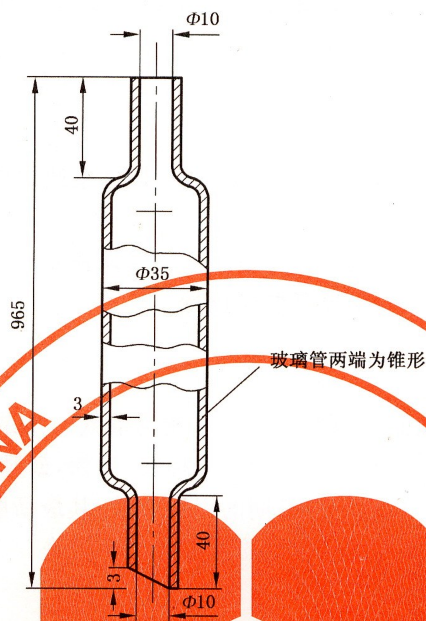
图 1 取样管
