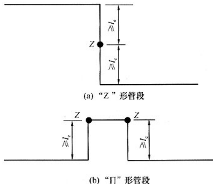
图4. 2. 4 转角管段布置示意图
