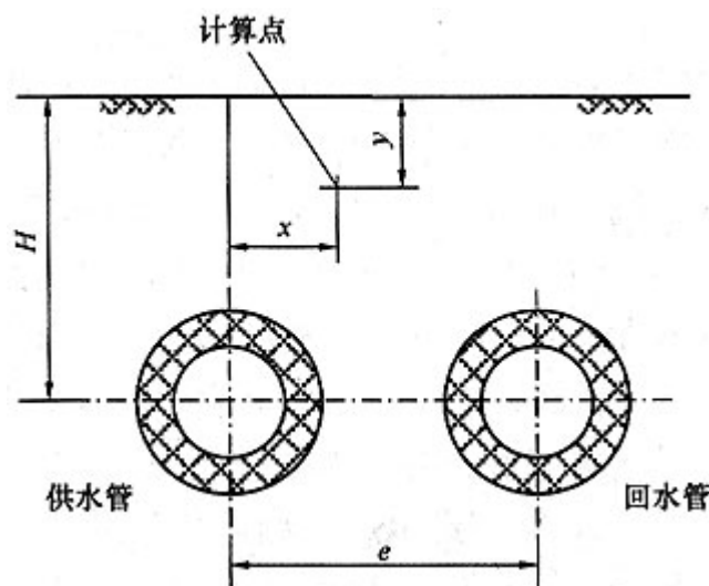
图1 保温计算示意图
