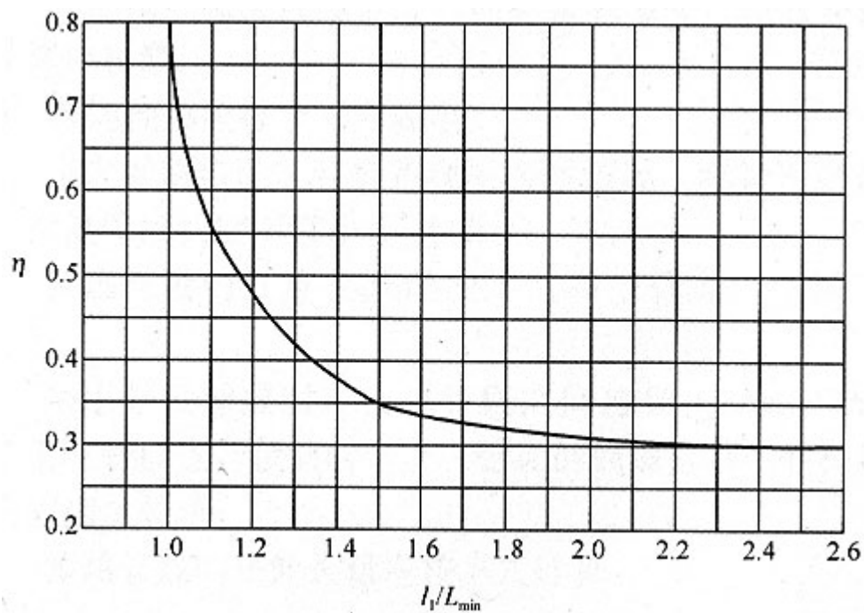
图D. 0. 3-2 综合抵消系数 \eta 曲线图
