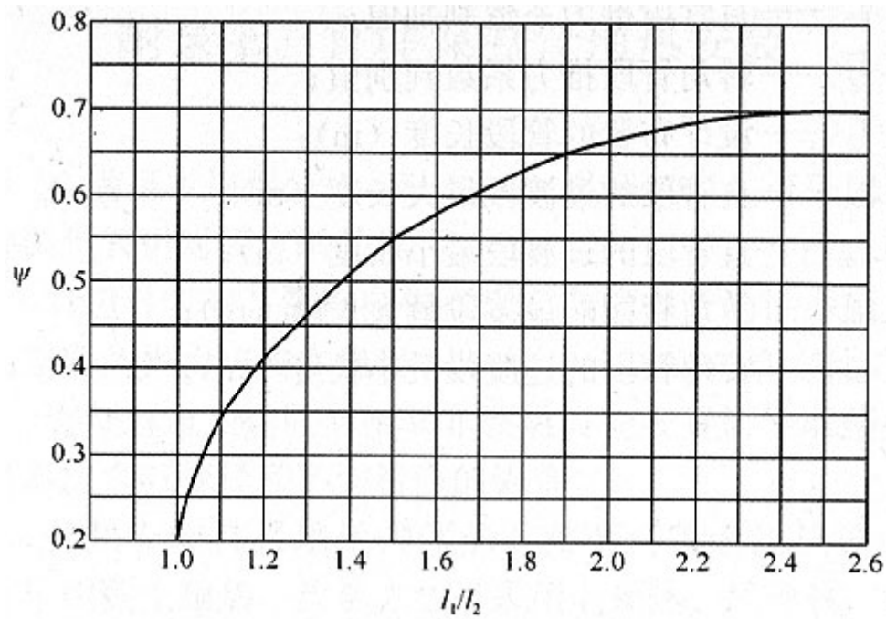
图D. 0. 3-1 推力系数 \Psi 曲线图
