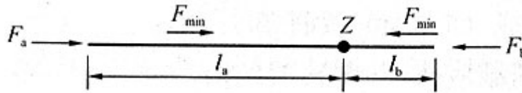
图5.7.1 计算驻点位置简图
