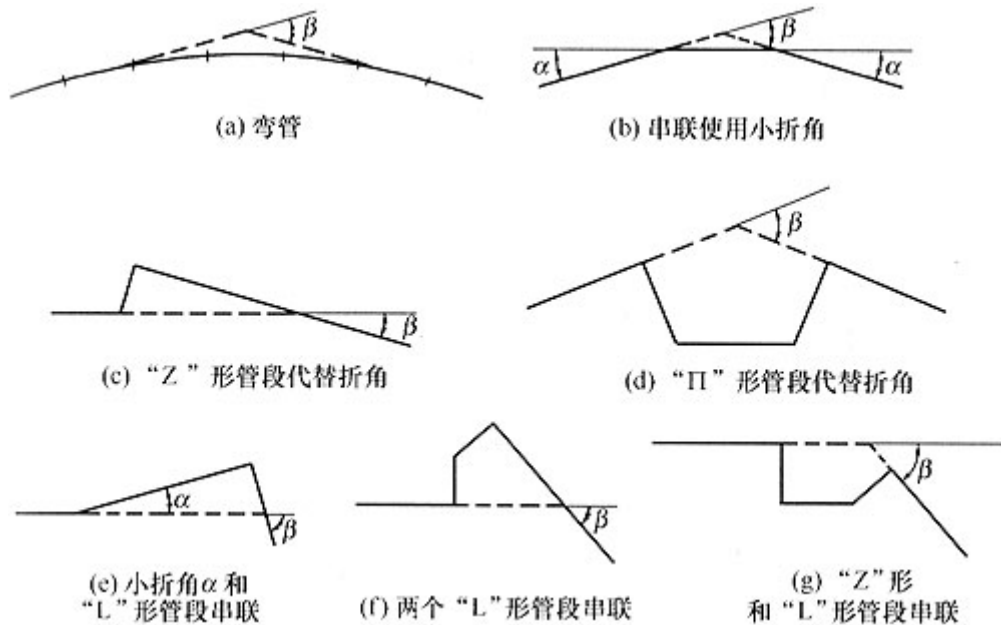
图4. 2. 6 管道的转角处理示意图
