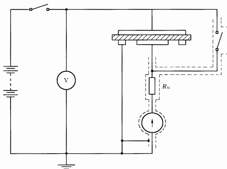
图 7 用作测量体积电阻的检流计法
