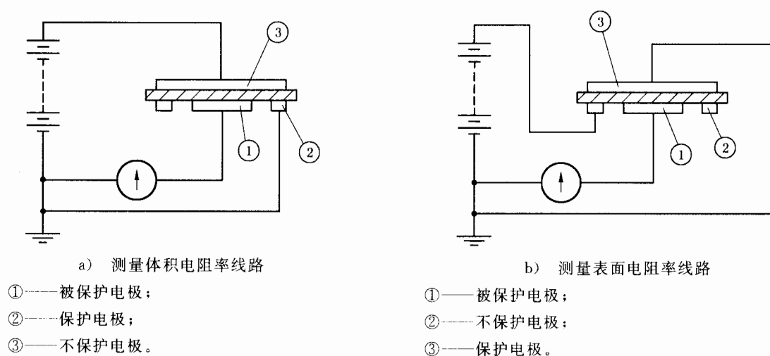
图 1 使用保护电极测量体积电阻率和表面电阻率的基本线路
