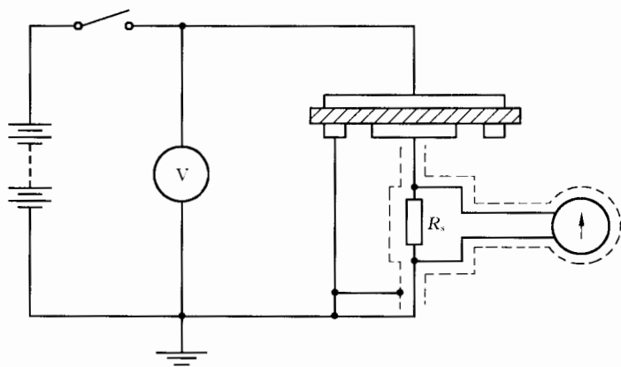
用作测量表面电阻时按图 1b) 联接试样 图 5 用来测量体积电阻的伏安法线路
