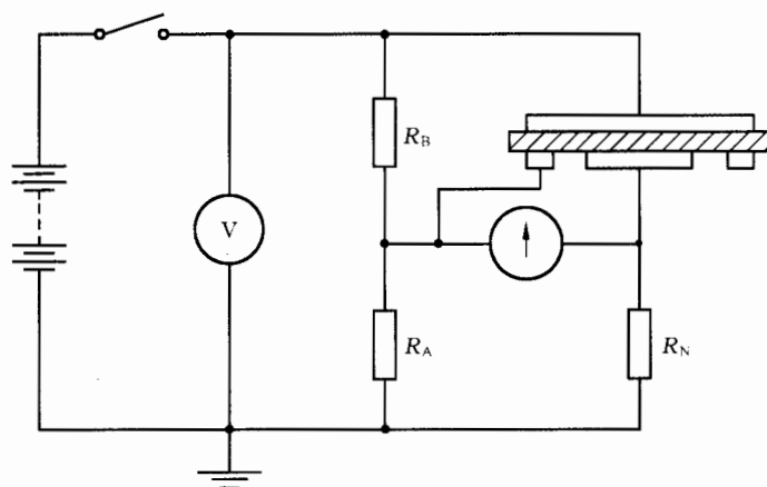
图 6 用于测量体积电阻的惠斯登电桥法
