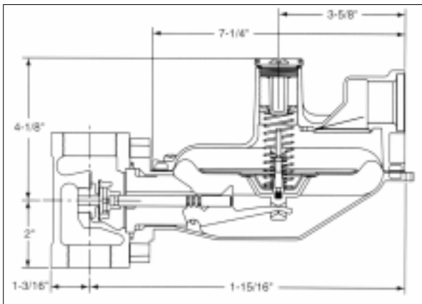
1813B2-HC-180° Dimensions
