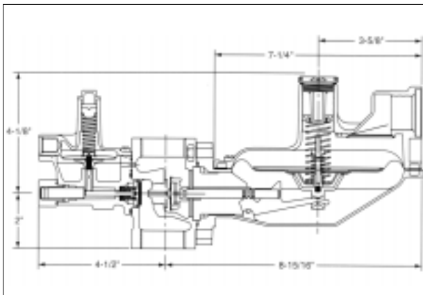
1843B2-HC Dimensions
