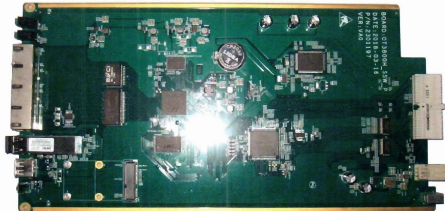
主控板
