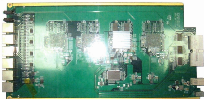
DSP 板
