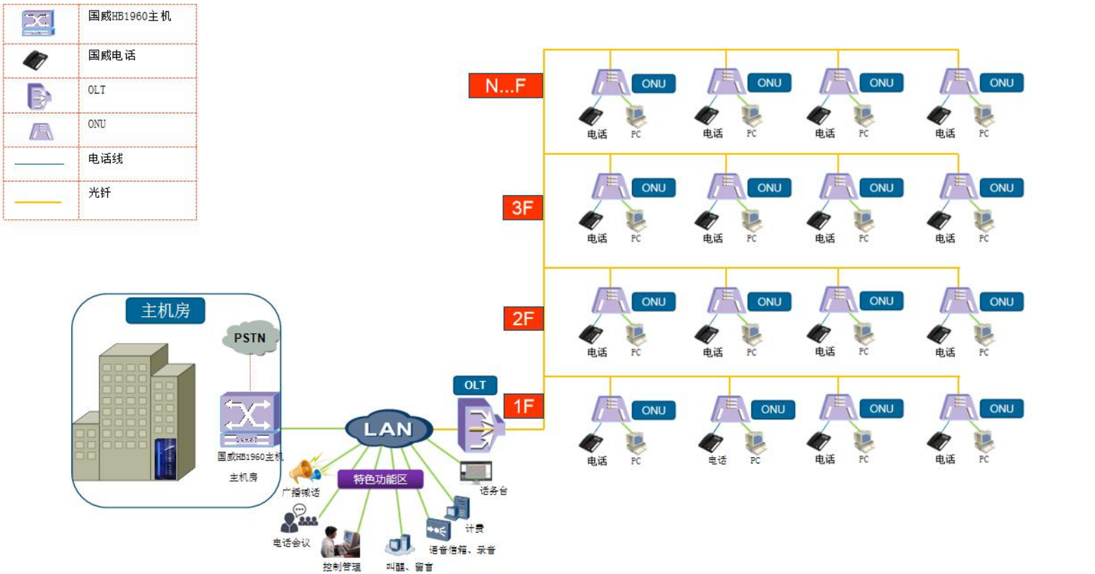
国威光通信拓扑图
