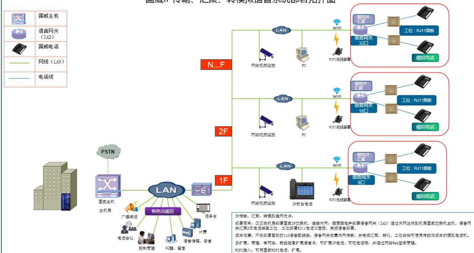
国威IP传输、汇聚、转模拟语音系统部署拓扑图
