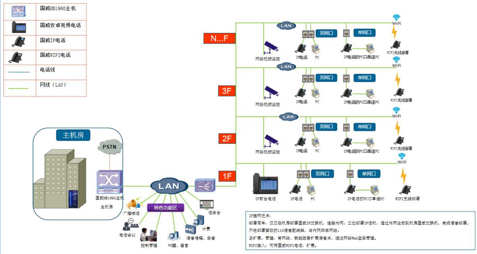
国威IP语音系统部署拓扑图
