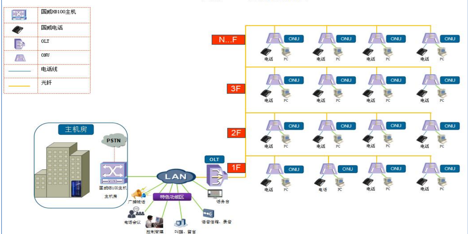
国威HB100光通信拓扑图
