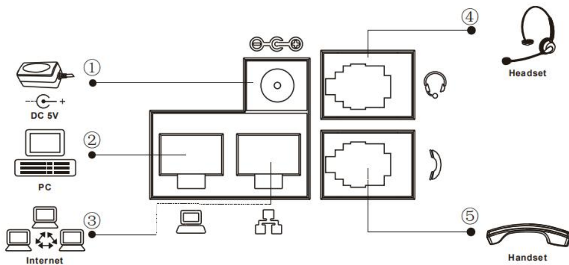
图 2 - 设备连接
