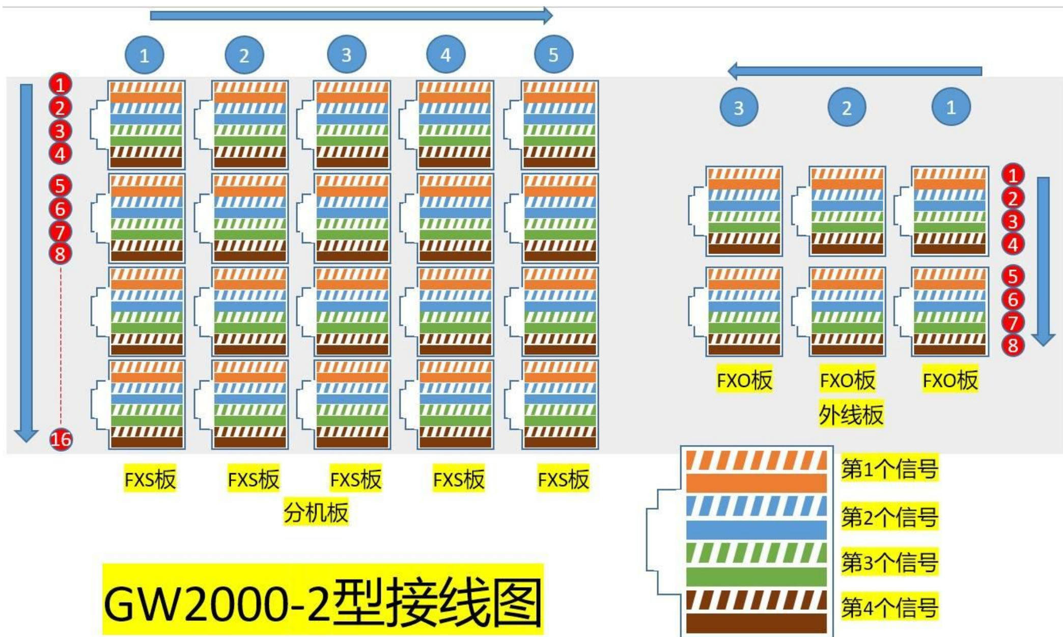
国威GW2000-2,板卡端口线序,接线图
