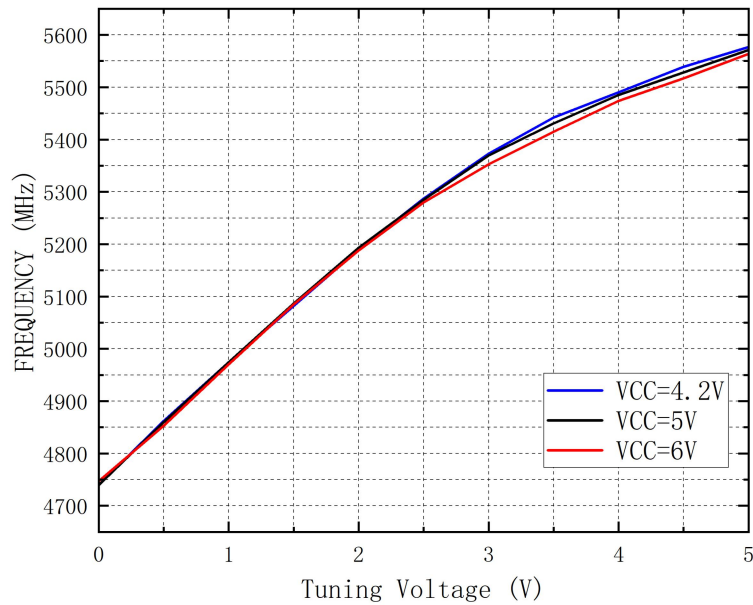
功率 vs. 调谐电压
