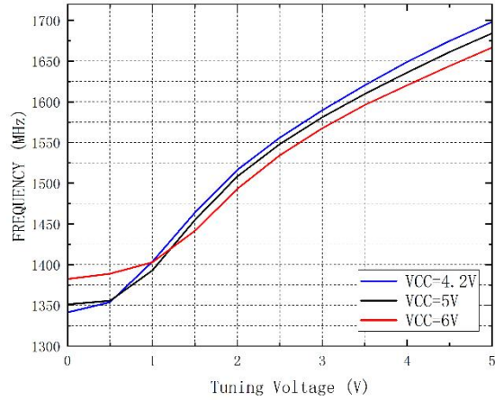
频率 vs.调谐电压vs.工作电压
