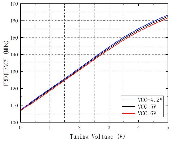
频率 vs.调谐电压vs.工作电压
