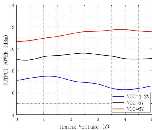
功率vs.调谐电压vs.VCC
