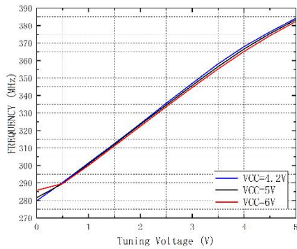
频率 vs. 调谐电压 vs. 工作电压
