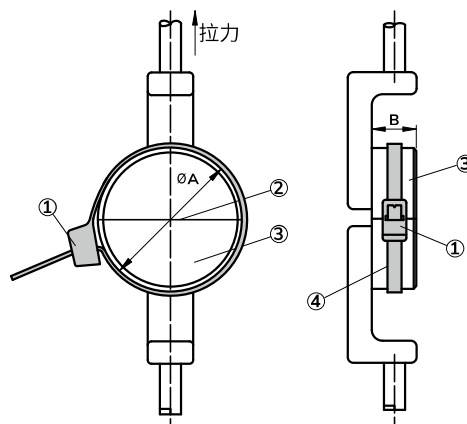
圖1.標準式紮線帶頭部需在左側
