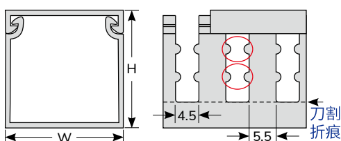
高度:80mm 雙凸點
