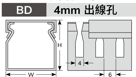
出線孔尺寸
