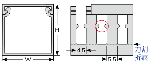
高度:60mm 單凸點
