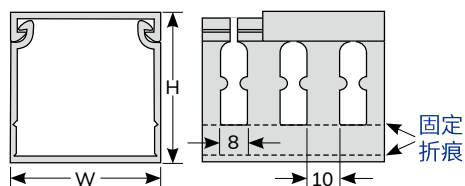
出線孔尺寸
