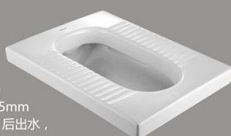
DT5003 蹲便器 尺寸：545x420x235mm 出水方式：带防臭，后出水，30孔距
