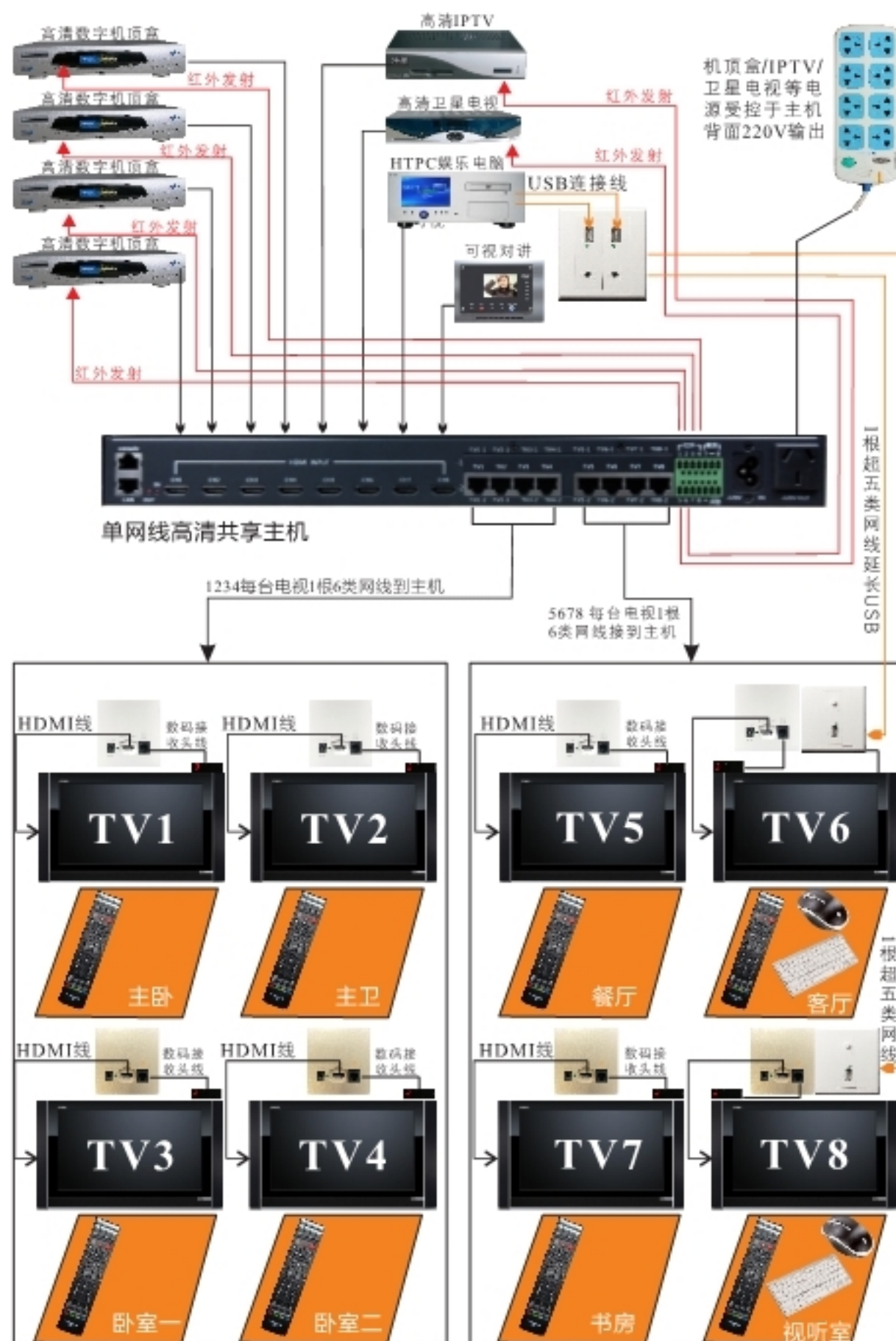
系统结构图
