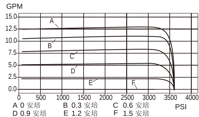
控制流量对应压力 油口3压力 > 油口2压力
