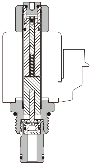
剖视图
