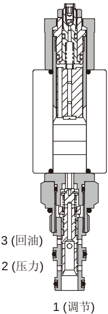
剖视图
