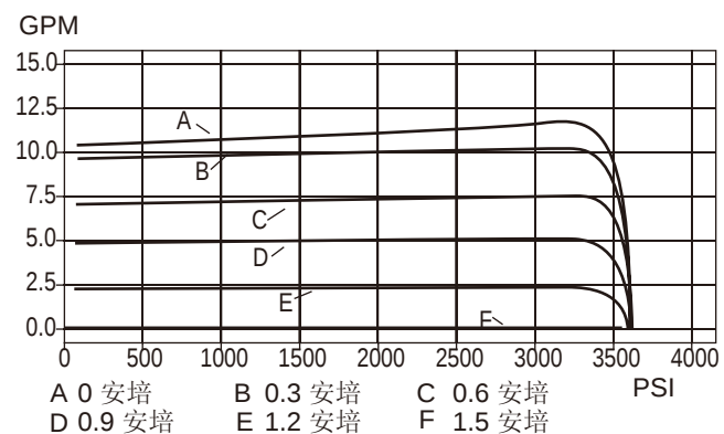
控制流量对应压力 油口2压力 > 油口3压力
