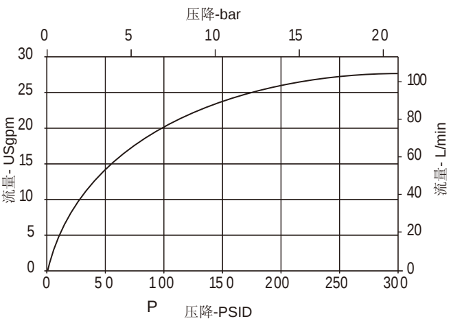
最大流量对应压降 流量额定值“B”(零电流)
