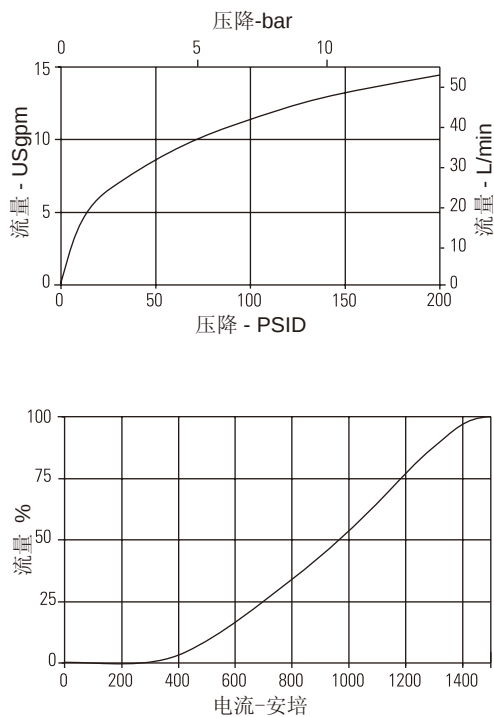
压降曲线
