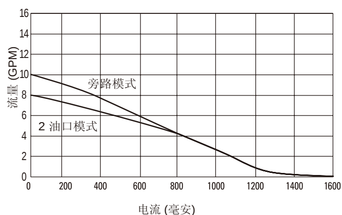
流量对应电流 - B 滑阀
