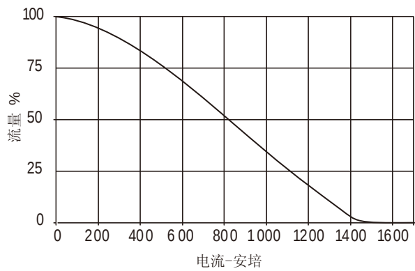
流量对应电流
