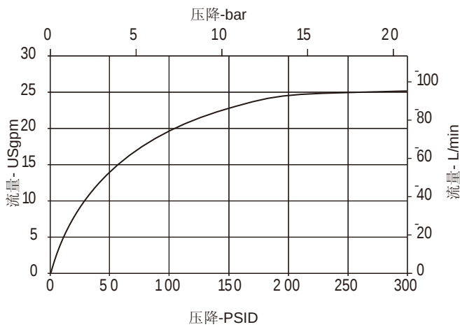
最大流量对应压降 流量额定值“A”(零电流)
