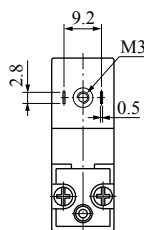
插座式 KGM215-D
