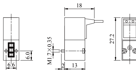
直接出线 KGM114
