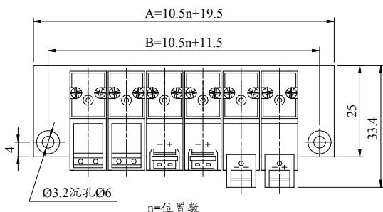
汇流板外形尺寸图 Manifold Dimensions (mm)
