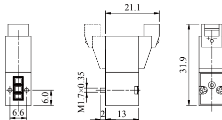
M型平行插座式 KGM114-M
