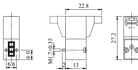
L型垂直插座式 KGM114-L
