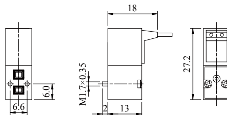
直接出线带自排型 KGM114-□-Z
