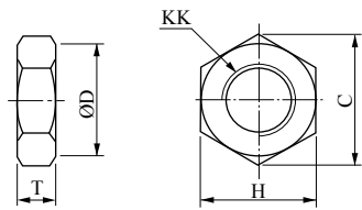
杆端螺母 (Rod End Nut)
