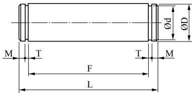
Y型肘节接头销子 (Knuckle Pin)
