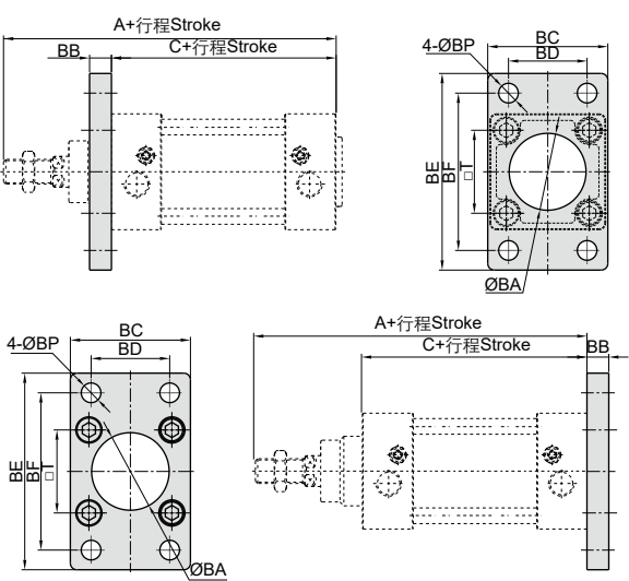
法兰Flange FA/FB
