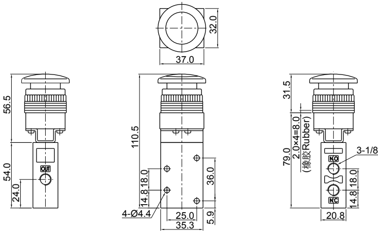
外形尺寸图 Dimensions (mm)
