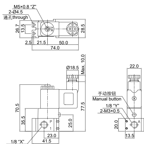
KSV111-D(DZ)/KSV112-D(DZ)
