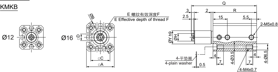
外形尺寸图 Dimensions (mm)
