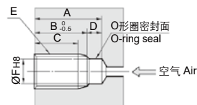
安装加工尺寸图 Machining dimensions for mounting
