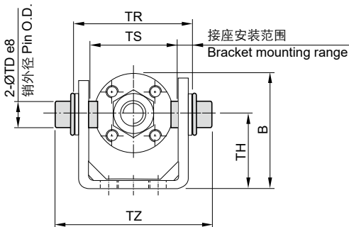
外形尺寸图 Dimensions (mm)
