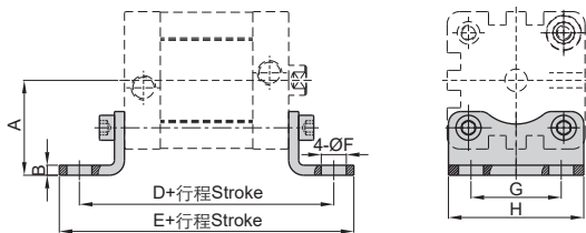
法兰Flange FNC
