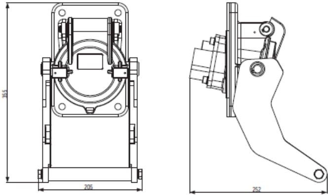
安装尺寸
