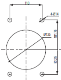
安装尺寸
