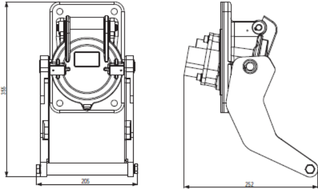
安装尺寸
