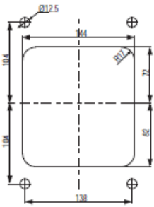
安装尺寸
