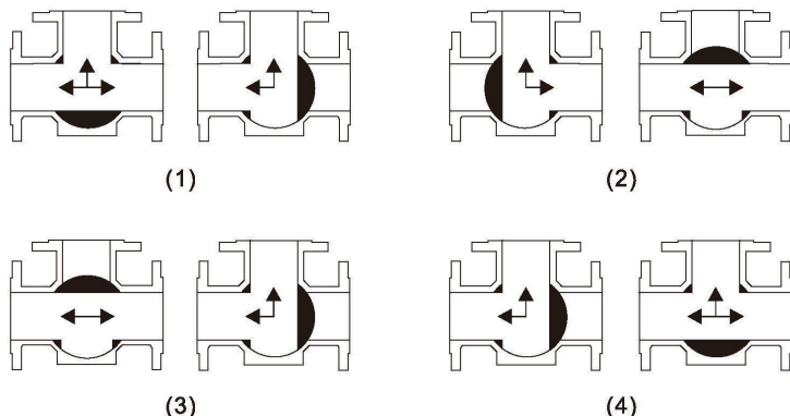
T型流向图
