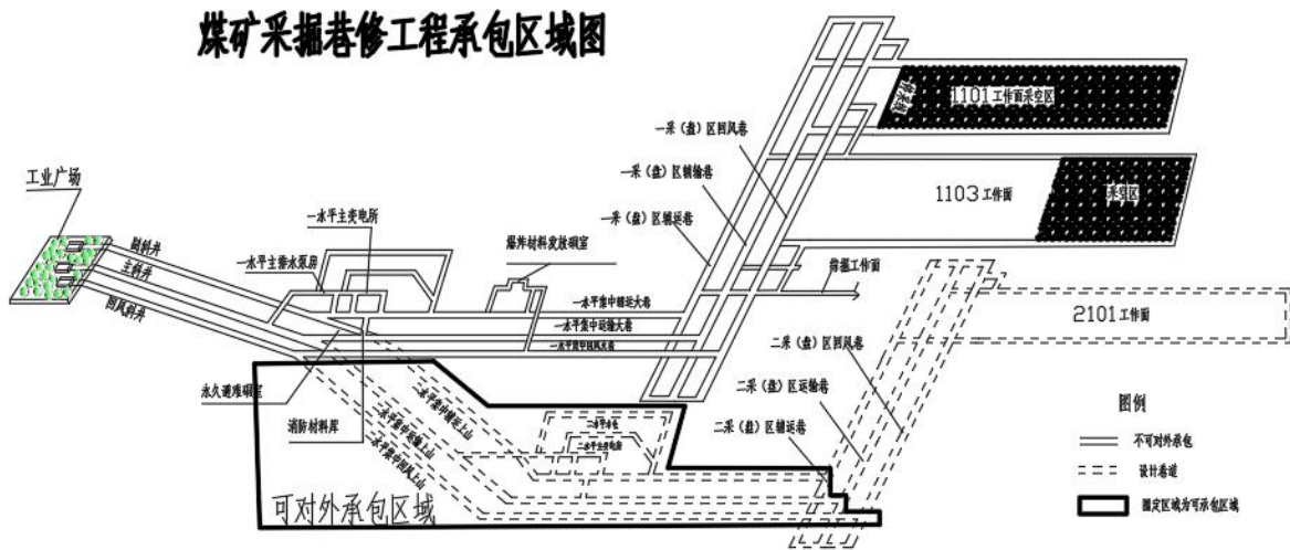
图 5 煤矿水平延深可独立承包的施工区域示意图
