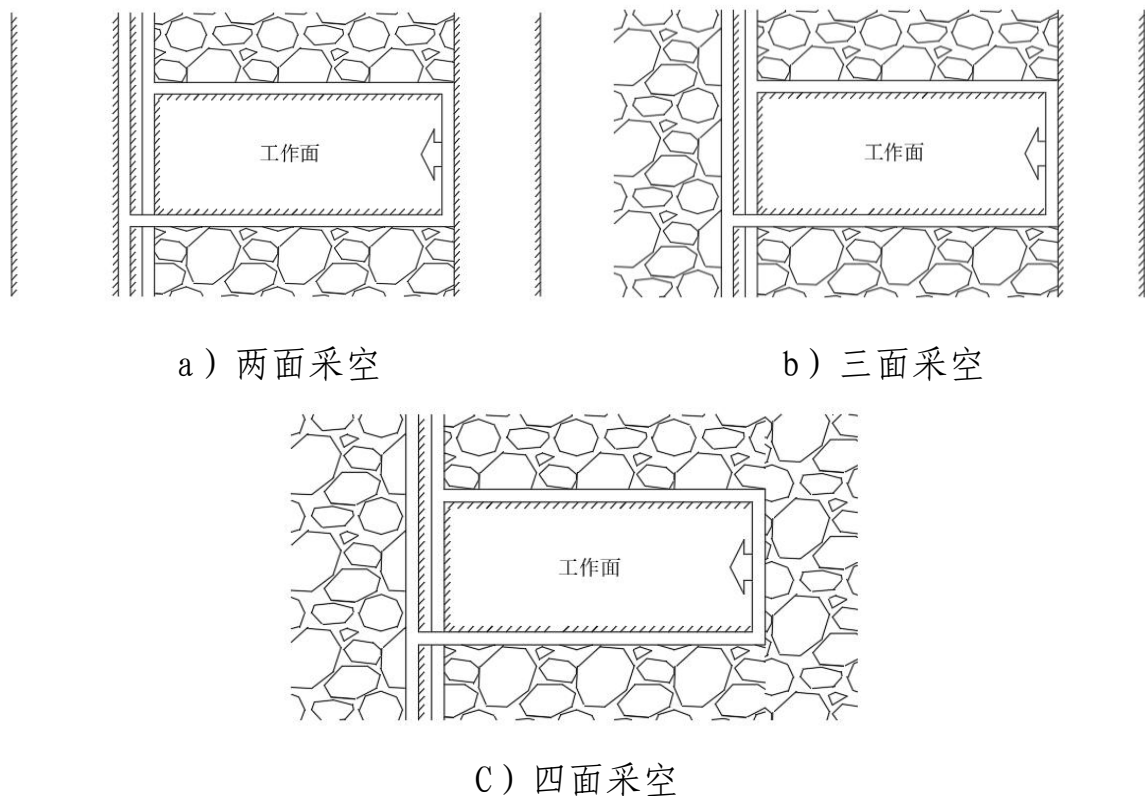
图 1 孤岛工作面（煤柱）示意图
