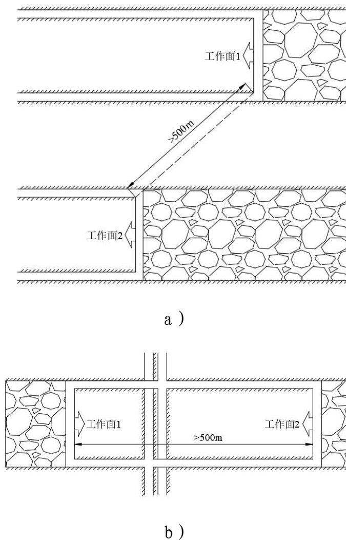
图 4 冲击地压危险煤层回采工作面距离要求
