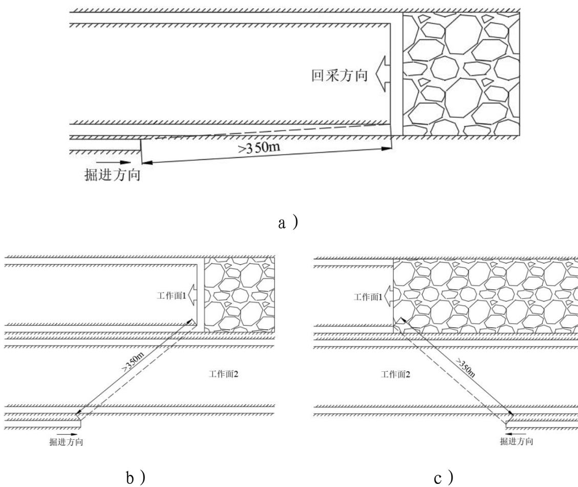
图 3 冲击地压危险煤层采掘工作面距离要求
