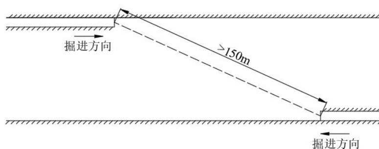
b) 不同巷道相向掘进
