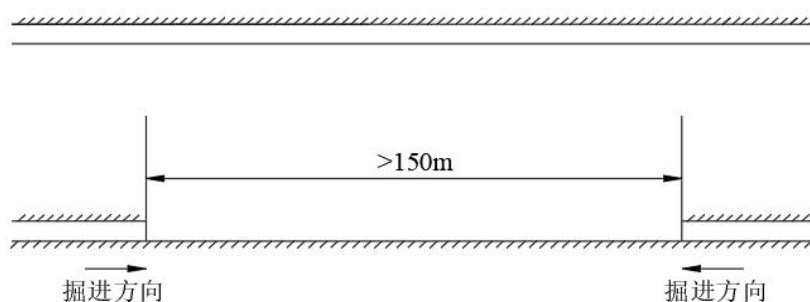
a) 同一巷道相向掘进
