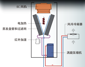
上送风-EC 风机
