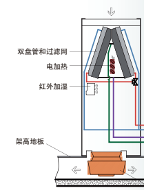
下送风-EC 风机
