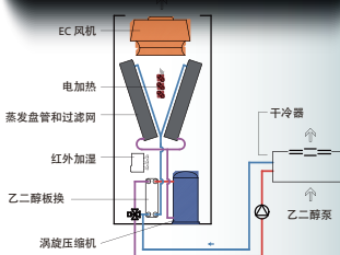
上送风-EC 风机
