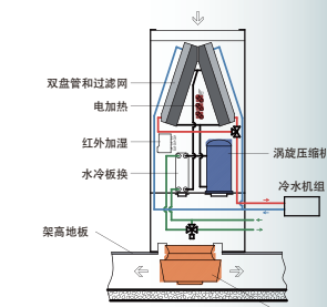
下送风-EC 风机
