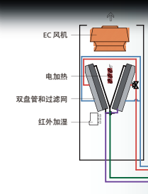
上送风-EC 风机
