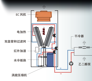
上送风-EC 风机
