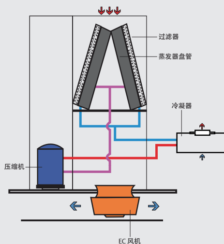
风冷/水冷下送风示意图
