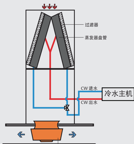
冷冻水下送风示意图
