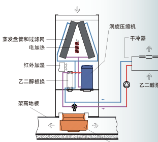
下送风-EC 风机
