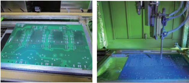
PCBA喷涂前蓝光检测 PCBA喷涂后蓝光检测
