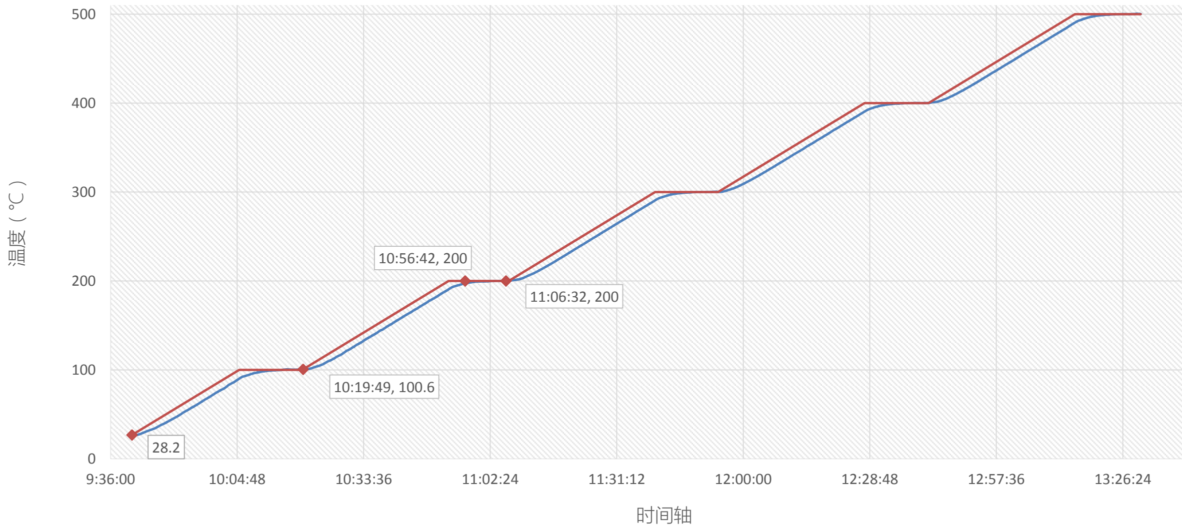
炉膛升温
