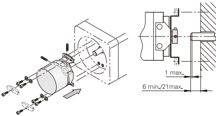
ERN 1123
