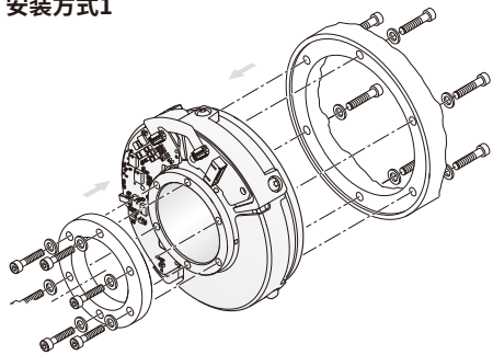
安装方式1
