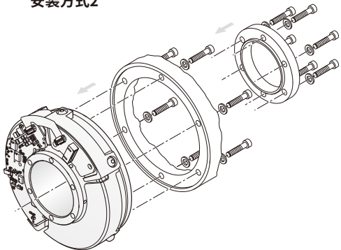
安装方式2
