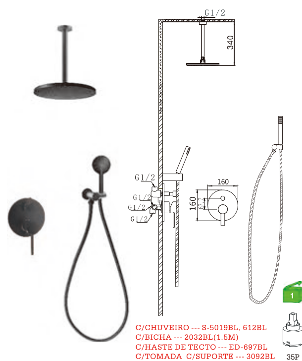
D26FK45BL Conj.Monocomando embutido 2 vias para duche Built-in shower mixer Conj.Monomando empotrado 2 vias para ducha 93.50€ (+IVA)
