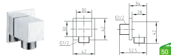
3091 Tomada de água Toma de agua 7.70€ (+IVA)
