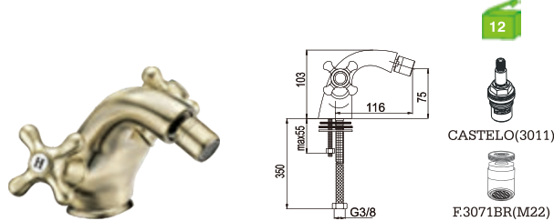
H15T4BR Misturadora bidé Bidet mixer Monobloc bidet
