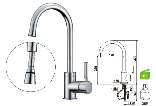
C30L7C C/bicha certificada Monocomando lava-loiça com chuveiro Kitchen mixer with pull out shower Monomando fregadero extraible 50.60€ BICHA ---2025(2M) (+IVA)
