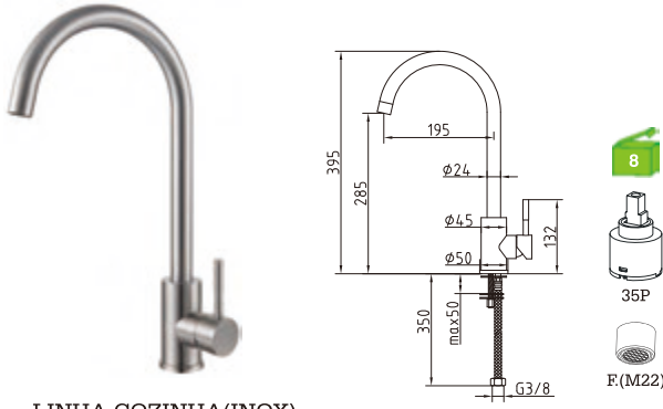
H30LA5C Monocomando de lava-loiça Kitchen mixer Monomando de fregadero
