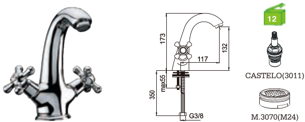
H15T1C Misturadora lavatório Basin mixer Monobloc lavabo
