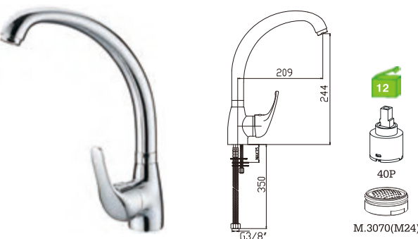
A68M18C Monocomando lava-loiça à banca bica alta Kitchen mixer Monomando fregadero (caño tubular)
