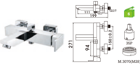
C53FX2C Monocomando banheira Bath/shower mixer Monomando banho C/CHUVEIRO---925 BICHA ---2031(1.7M) SUPORTE ---KH INVERSOR ---3035
