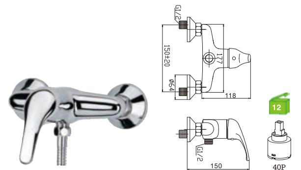
A68M3C Monocomando duche Shower mixer Monomando ducha
