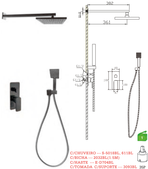
D21RP47BL Conj.Monocomando embutido 2 vias para duche Built-in shower mixer Conj.Monomando empotrado 2 vias para ducha 110.00€ (+IVA)
