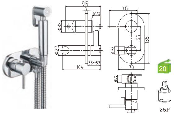
L12CB4C Misturadora de Torneira para bidê/WC, abertura 90°. Chuveiro em latão Tap for bidet/toilets, 90° opening. Brass handshower Grifo para bidé/WC, abertura 90°. Ducha en latón 37.50€ (+IVA)
