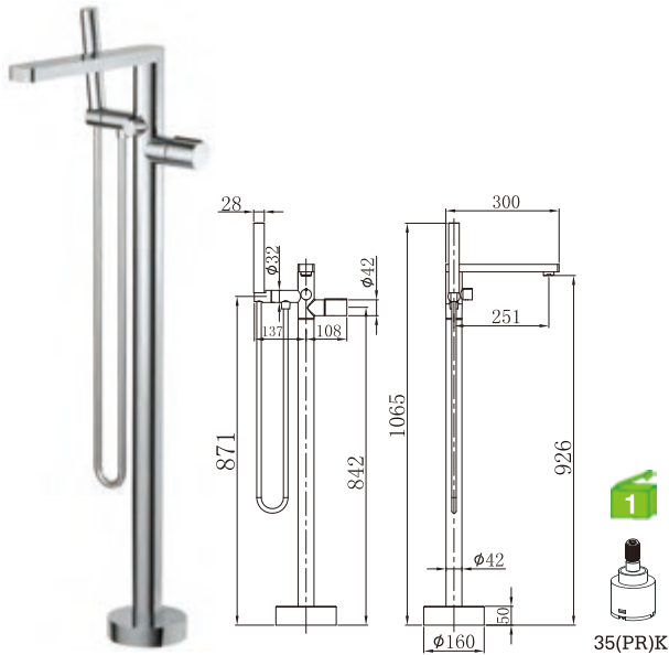
D25WR25C Monocomando de banheira e duche, montagem ao chão Single-lever bath/shower mixer, floor-mounted Monomando para baño y ducha de pie 234.00€ (+IVA)
