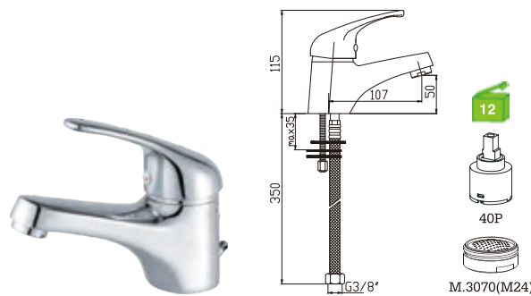
A68M1C Monocomando lavatório Basin mixer Monomando lavabo
