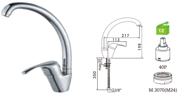
C15DF8C Monocomando lava-loiça à banca bica alta Kitchen mixer Monomando fregadero (caño tubular) C/bicha certificada 19.20€ (+IVA)
