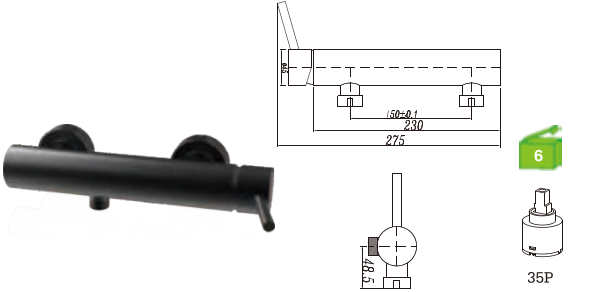
E34GP3BL Monocomando duche Shower mixer Monomando ducha CHUVEIRO ---612BL BICHA ---2032BL(1.5M) SUPORTE ---PH(BL) 53.50€ (+IVA)
