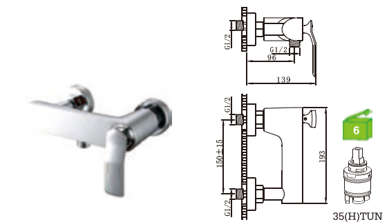
E38BS3C Monocomando duche Shower mixer Monomando ducha
