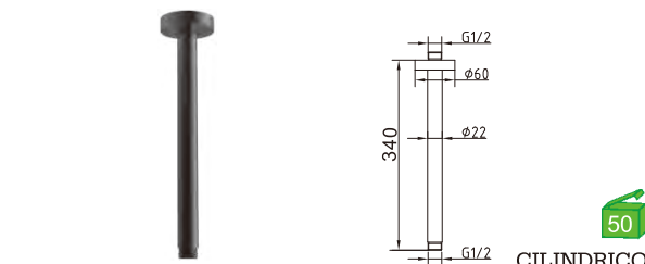
ED-697BL Haste de tecto Barra de pared 9.00€ (+IVA)
