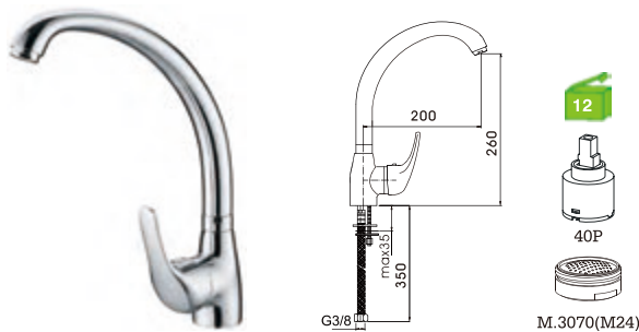
C17DF8C Monocomando lava-loiça à banca bica alta Kitchen mixer Monomando fregadero (caño tubular) C/bicha certificada 21.00€ (+IVA)
