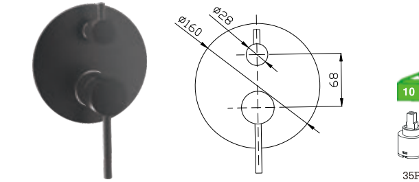
D26FK42BL(B) Monocomando embutido 2 vias Built-in mixer Monomando empotrado 2 vias 52.50€ (+IVA)
