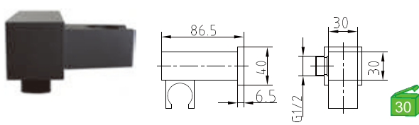
3093BL Tomada de água com suporte Toma de agua con soporte 17.50€ (+IVA)
