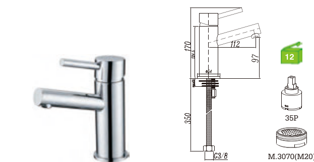
E34GP1C-1 Monocomando lavatório Basin mixer Monomando lavabo
