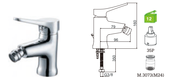
C38DA4C Monocomando bidé Bidet mixer Monomando bidet
