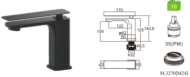
D22HB1BL-1 Monocomando lavatório Basin mixer Monomando lavabo C/bicha certificada 45.00€ (+IVA)
