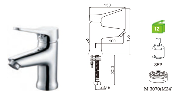
C38DA1C Monocomando lavatório Basin mixer Monomando lavabo
