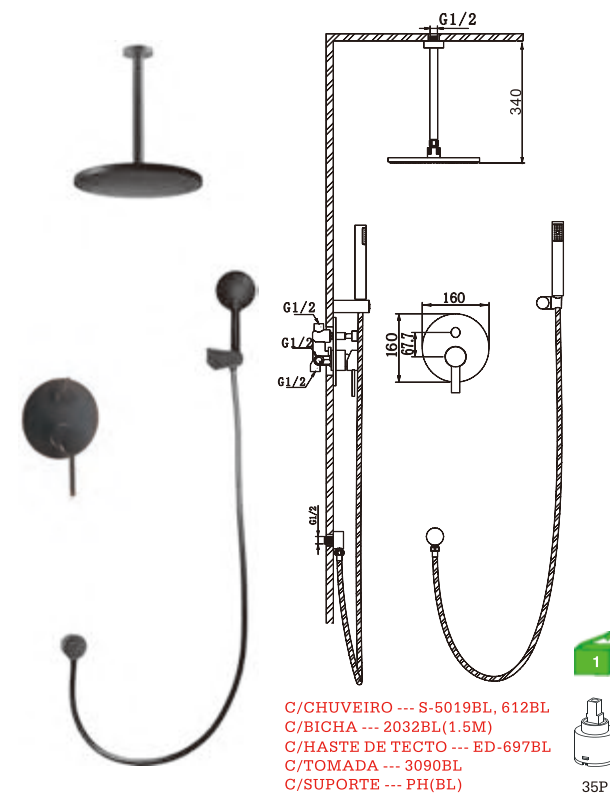
D26FK46BL Conj.Monocomando embutido 2 vias para duche Built-in shower mixer Conj.Monomando empotrado 2 vias para ducha 85.50€ (+IVA)
