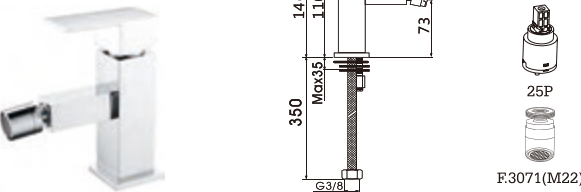
C53FD4C Monocomando bidé Bidet mixer Monomando bidet
