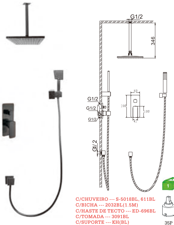
D21RP45BL Conj.Monocomando embutido 2 vias para duche Built-in shower mixer Conj.Monomando empotrado 2 vias para ducha 97.30€ (+IVA)
