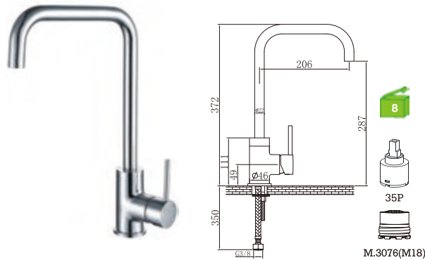
C45GB18C Monocomando lava-loiça Kitchen mixer Monomando fregadero
