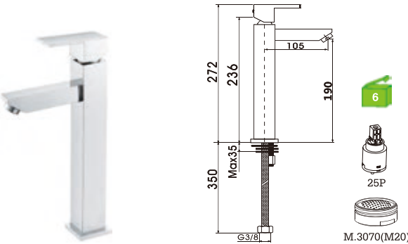
C53FD1C Monocomando lavatório alto Basin mixer Monomando lavabo alto
