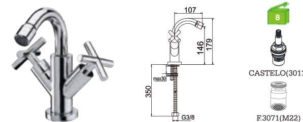
C30X4C Misturadora bidé Bidet mixer Monobloc bidet
