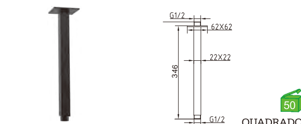
ED-696BL Haste de tecto Barra de pared 14.50€ (+IVA)
