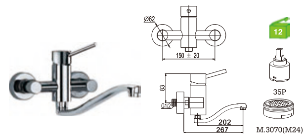
E34GP6C Monocomando lava-loiça à parede bica baixa Wall mounted kitchen mixer Monomando Fregadero pared (caño baixo) BICA ---3060
