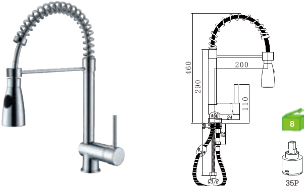
C35GK17C Monocomando de lava-loiça industrial Industry kitchen mixer Monomando de fregadero industrial C/CHUVEIRO---161 BICHA ---2024
