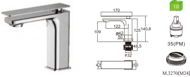
D22HB1C-1 Monocomando lavatório Basin mixer Monomando lavabo C/bicha certificada 40.00€ (+IVA)
