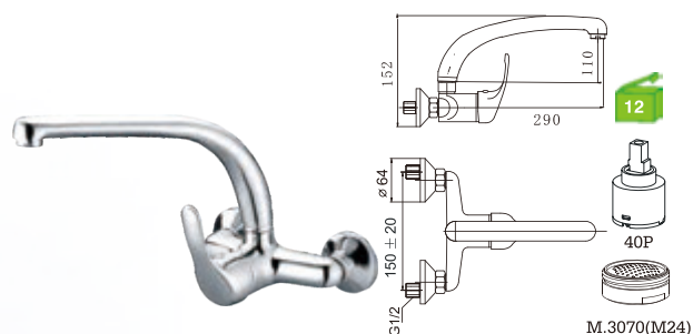
R26M19C Monocomando lava-loiça à parede bica alta-fundida Wall mounted kitchen mixer Monomando fregadero pared (caño fundido) BICA ---3061
