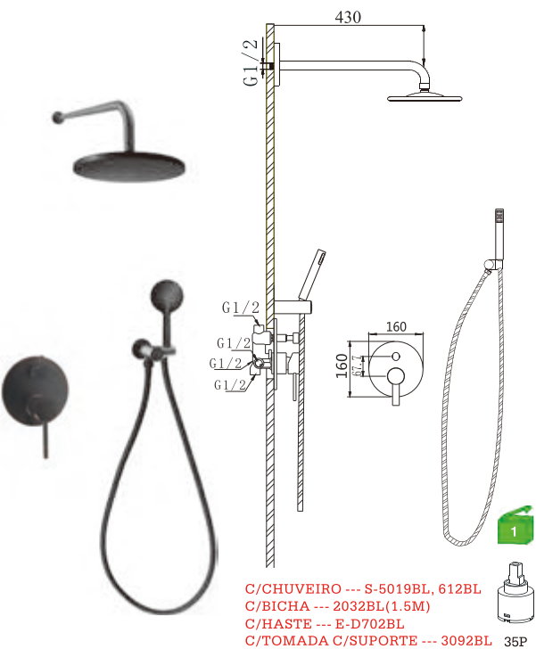
D26FK44BL Conj.Monocomando embutido 2 vias para duche Built-in shower mixer Conj.Monomando empotrado 2 vias para ducha 92.50€ (+IVA)
