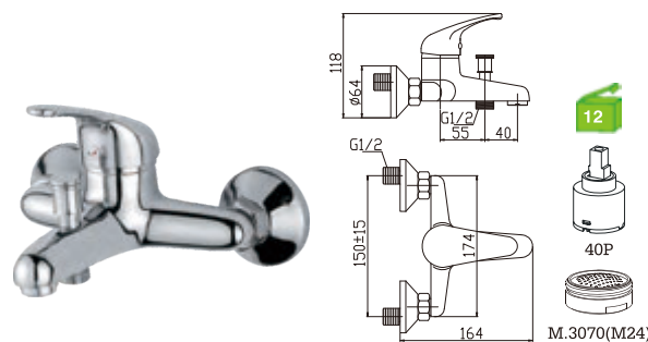
A68M2C Monocomando banheira Bath/shower mixer Monomando baño
