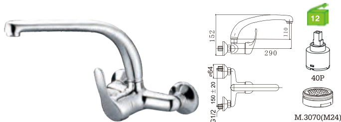
C17DF9C Monocomando lava-loiça à parede bica alta-fundida Wall mounted kitchen mixer Monomando fregadero pared (caño fundido) BICHA ---3061 36.20€ (+IVA)
