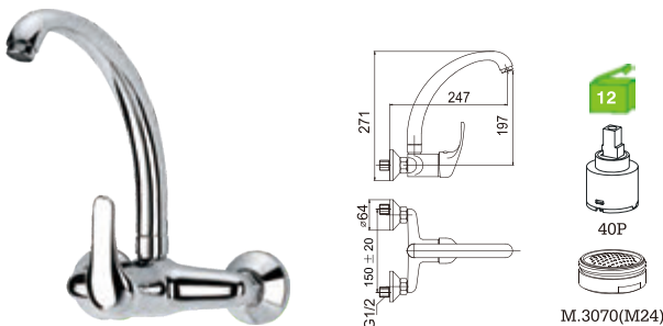
C15DF9C Monocomando lava-loiça à parede bica alta Wall mounted kitchen mixer Monomando fregadero pared (caño alto) BICHA ---3064 25.50€ (+IVA)
