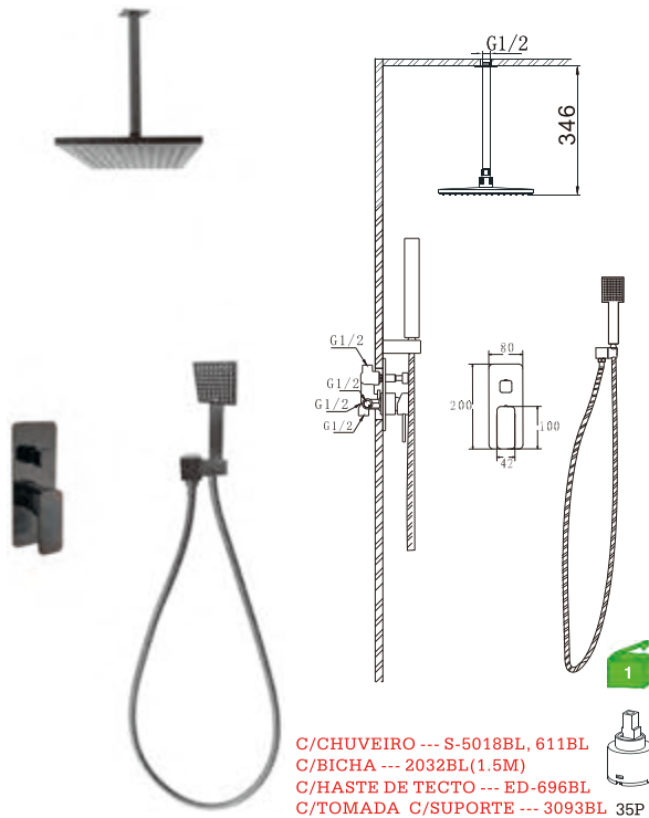
D21RP46BL Conj.Monocomando embutido 2 vias para duche Built-in shower mixer Conj.Monomando empotrado 2 vias para ducha 103.00€ (+IVA)
