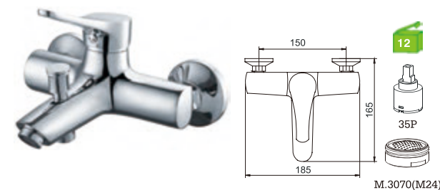
C38DA2C Monocomando banheira Bath/shower mixer Monomando baño C/CHUVEIRO ---168 BICHA ---2031(1.7M) SUPORTE ---JH INVERSOR ---3030
