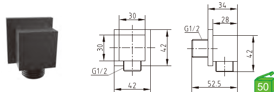
3091BL Tomada de água Toma de agua 10.00€ (+IVA)
