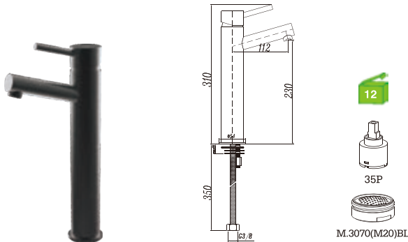
E34GP1BL Monocomando lavatório alto Basin mixer Monomando lavabo alto C/bicha certificada S/VÁLVULA 43.10€ (+IVA)
