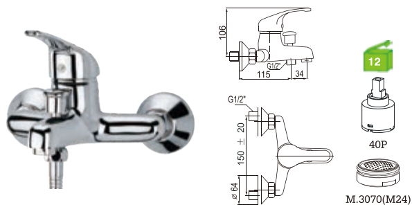
C15DF2C Monocomando banheira Bath/shower mixer Monomando baño C/CHUVEIRO---168 BICHA ---2031(1.7M) SUPORTE ---JH INVERSOR ---3030 29.20€ (+IVA)
