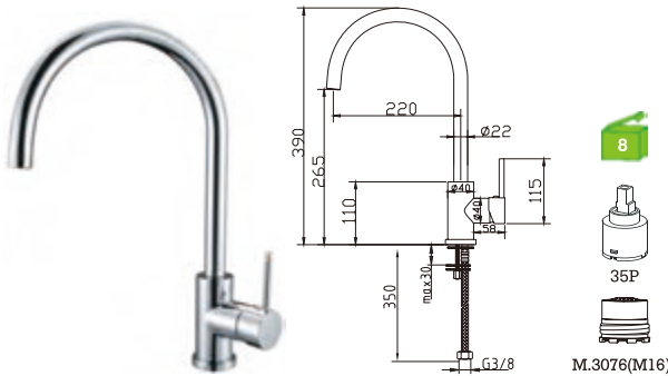
E37GB5C Monocomando de lava-loiça Kitchen mixer Monomando de fregadero
