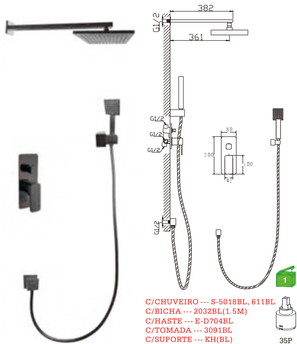
D21RP44BL Conj.Monocomando embutido 2 vias para duche Built-in shower mixer Conj.Monomando empotrado 2 vias para ducha 105.00€ (+IVA)
