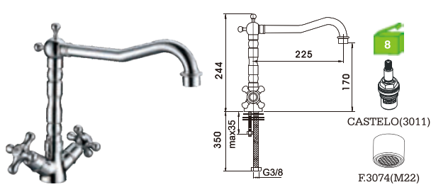
H15T15C Misturadora lava-loiça Kitchen mixer Monobloc fregadero
