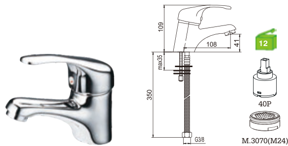
C15DF1C Monocomando lavatório Basin mixer Monomando lavabo C/bicha certificada S/VALVULA 17.60€ (+IVA)
