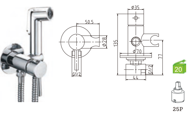
L11CA4C Misturadora de encastrar para bidê/WC. Chuveiro em ABS - EloR Concealed single lever mixer bidet/toilets. ABS hand shower - EloR Mezclador de empotrar para bidé/WC. Ducha en ABS - EloR 30.00€ (+IVA)
