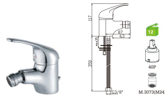
A68M4C Monocomando bidé Bidet mixer Monomando bidet
