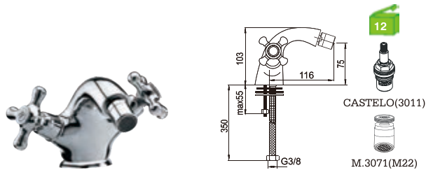
H15T4C Misturadora bidé Bidet mixer Monobloc bidet
