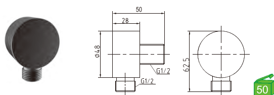
3090BL Tomada de água Toma de agua 6.80€ (+IVA)
