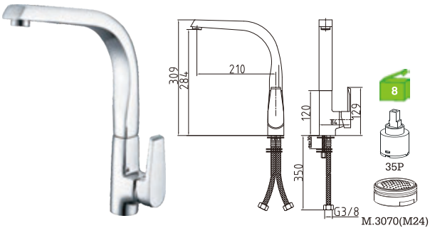
E37GM8C Monocomando lava-loiça Kitchen mixer Monomando fregadero
