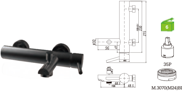
E34GP2BL Monocomando banheira Bath/shower mixer Monomando baño CHUVEIRO ---612BL BICHA ---2032BL(1.5M) SUPORTE ---PH(BL) INVERSOR ---3037BL 65.00€ (+IVA)
