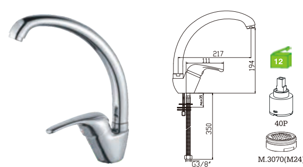
A68M8C Monocomando lava-loiça à banca bica alta Kitchen mixer Monomando fregadero (caño tubular)
