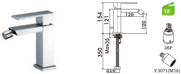
C51FT4C Monocomando bidet Bidet mixer Monomando bidet
