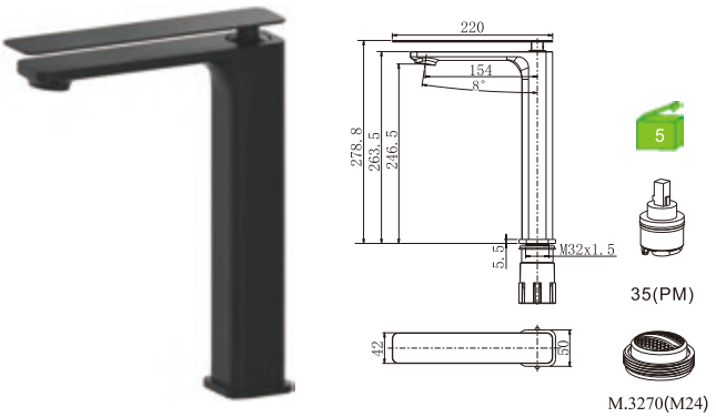
D22HK1BL Monocomando lavatório alto Basin mixer Monomando lavabo alto C/bicha certificada 76.30€ (+IVA)
