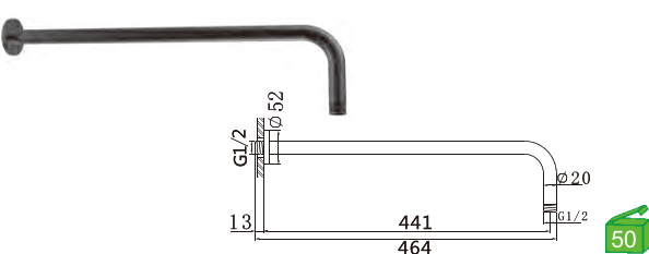
E-D702BL Haste de parede Barra de pared 8.30€ (+IVA)
