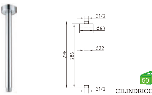
ED-697 Haste de tecto Barra de techo 7.50€ (+IVA)
