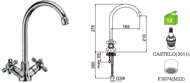
H15T5C Misturadora lava-loiça Kitchen mixer Monobloc fregadero BICA ---3068
