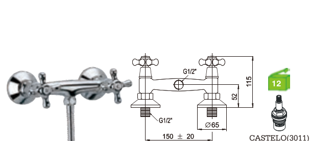
H15T3C Misturadora duche Shower mixer Monobloc ducha C/CHUVEIRO---888CR BICHA ---2031(1.7M) SUPORTE ---MH
