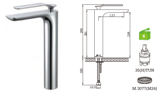
E38BK1C Monocomando lavatório alto Basin mixer Monomando lavabo alto
