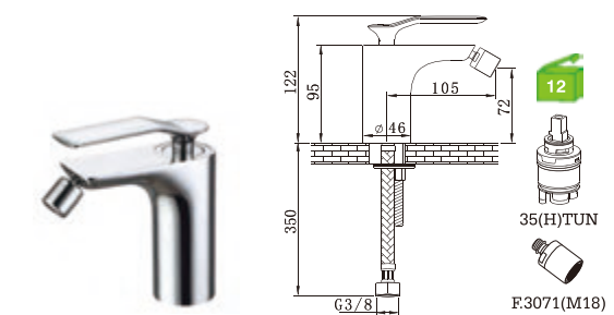
E38BS4C Monocomando bidé Bidet mixer Monomando bidet
