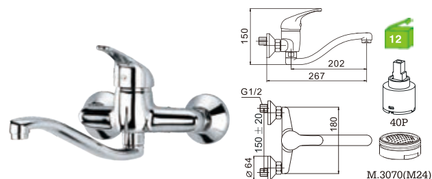
R26M6C Monocomando lava-loiça à parede bica baixa Wall mounted kitchen mixer Monomando fregadero pared (caño baixo) BICA ---3060
