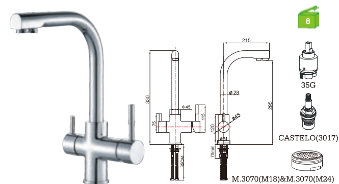
C30L8C C/bicha certificada Monocomando lava-loiça dupla função da água purificada Kitchen mixer double function – purified water Monomando fregadero doble función – agua depurada 69.00€ (+IVA)
