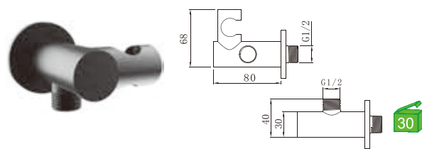
3092BL Tomada de água com suporte Toma de agua con soporte 16.30€ (+IVA)
