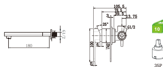
D21RP10BL Monocomando lavatório embutido In wall basin mixer Monomando lavabo empotrado
