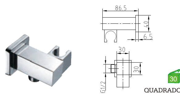
3093 Tomada de água com suporte Toma de agua con soporte 16.30€ (+IVA)
