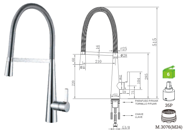
E36GH17C C/bicha certificada Monocomando de lava-loiça industrial Industry kitchen mixer Monomando de fregadero industrial 79.00€ (+IVA)
