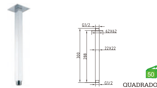
ED-696 Haste de tecto Barra de techo 12.20€ (+IVA)
