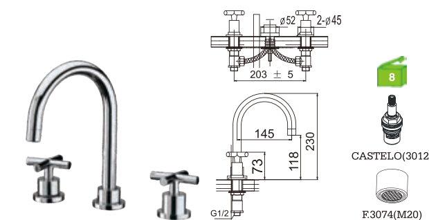
C30X10C Misturadora lavatório 3 furos Basin mixer Monobloc lavabo
