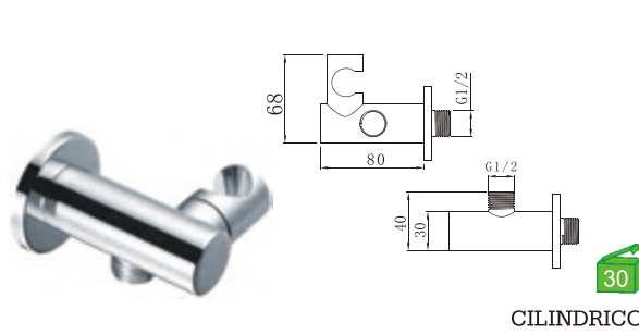
3092 Tomada de água com suporte Toma de agua con soporte 15.00€ (+IVA)
