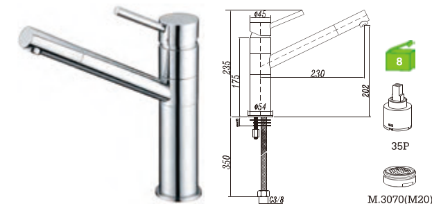
E34GP5C Monocomando lava-loiça Kitchen mixer Monomando fregadero
