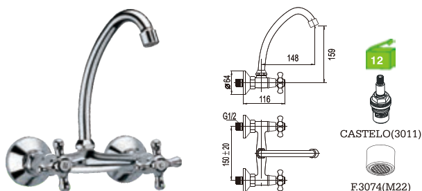
H15T9C Misturadora lava-loiça à parede bica alta Wall mouted kitchen mixer Monobloc fregadero pared (caño alto) BICA ---3062
