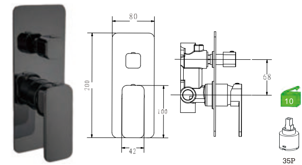
D21RP42BL(B) Monocomando embutido 2 vias Built-in mixer Monomando empotrado 2 vias 52.50€ (+IVA)
