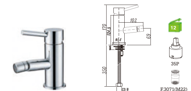
E34GP4C Monocomando bidé Bidet mixer Monomando bidet
