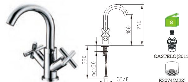
C36X1C-1 Misturadora lavatório Basin mixer Monobloc lavabo
