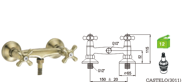
H15T3BR Misturadora duche Shower mixer Monobloc ducha C/CHUVEIRO---888BR BICHA ---2030BR(1.7M) SUPORTE ---MH(BR)
