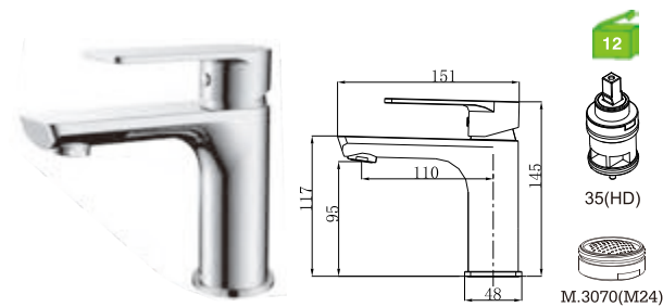
E22BH1C-1 Monocomando lavatório Basin mixer Monomando lavabo
