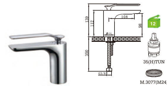
E38BK1C-1 Monocomando lavatório Basin mixer Monomando lavabo
