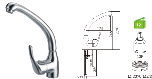
C16DF8C Monocomando lava-loiça à banca bica alta-fundida Kitchen mixer Monomando fregadero (caño fundido) C/bicha certificada 32.80€ (+IVA)
