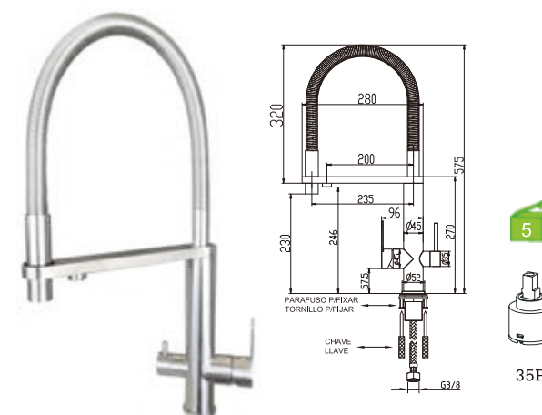
H30LP8X Monocomando lava-loiça dupla função da água purificada industrial Kitchen mixer double function – purified water Monomando fregadero doble función – agua Ósmosis industrial
