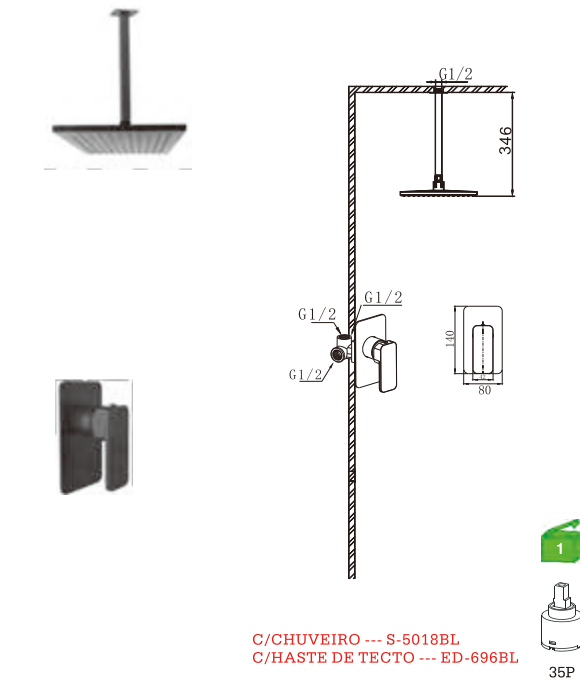
D21RP33BL Monocomando embutido 1 via Built-in mixer Monomando empotrado 1 via 60.80€ (+IVA)
