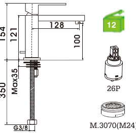
C51FX28C Monocomando lava-loiça dupla função da água purificada Kitchen mixer double function – purified water Monomando fregadero doble función – agua depurada
