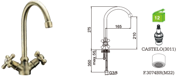
H15T5BR Misturadora lava-loiça Kitchen mixer Monobloc fregadero BICA ---3068(BR)
