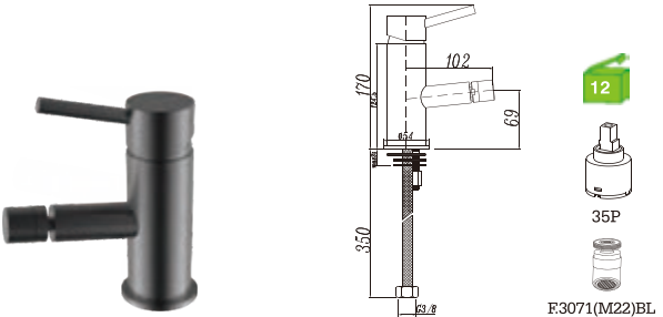
E34GP4BL Monocomando bidé Bidet mixer Monomando bidet C/bicha certificada S/VÁLVULA 34.00€ (+IVA)
