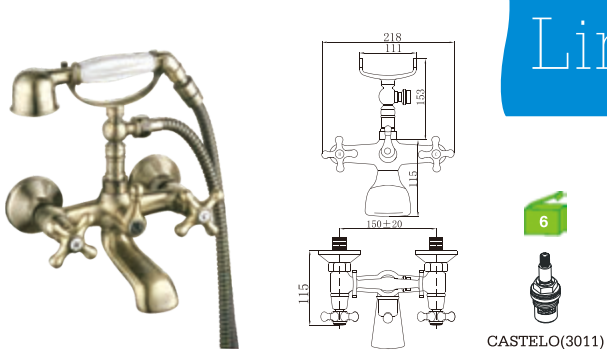
H15T2BR Misturadora banheira Bath/shower mixer Monobloc baño C/CHUVEIRO---888BR BICHA ---2030BR(1.7M) SUPORTE ---MH(BR)
