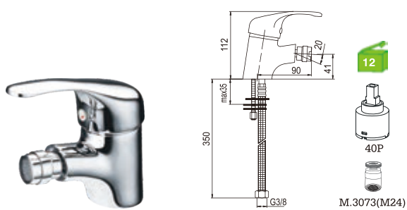
C15DF4C Monocomando bidé Bidet mixer Monomando bidet C/bicha certificada S/VALVULA 17.60€ (+IVA)
