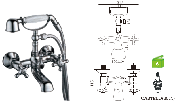
H15T2C Misturadora banheira Bath/shower mixer Monobloc baño C/CHUVEIRO---888CR BICHA ---2031(1.7M) SUPORTE ---MH
