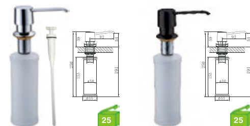
5066 Doseador de plástico
