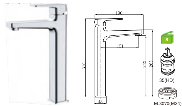
E21BF1C Monocomando lavatório alto Basin mixer Monomando lavabo alto
