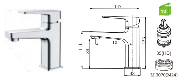
E21BF1C-1 Monocomando lavatório Basin mixer Monomando lavabo
