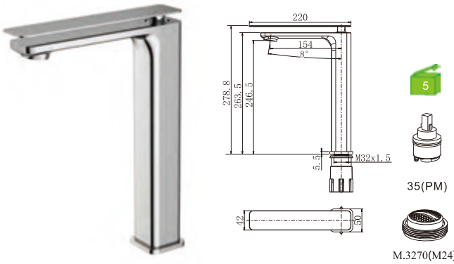
D22HK1C Monocomando lavatório alto Basin mixer Monomando lavabo alto C/bicha certificada 67.50€ (+IVA)
