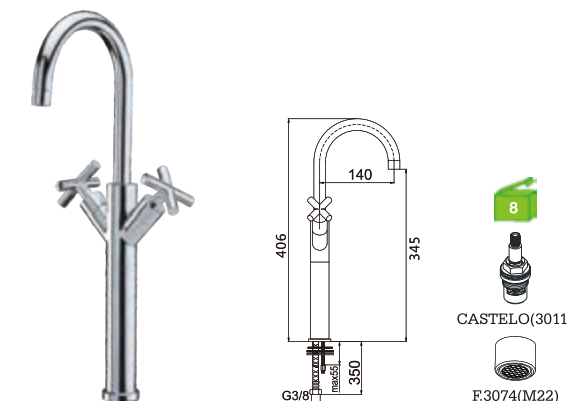
C36X1C Misturadora lavatório alto Basin mixer Monobloc lavabo alto
