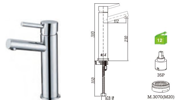
E34GP1C Monocomando lavatório alto Basin mixer Monomando lavabo alto
