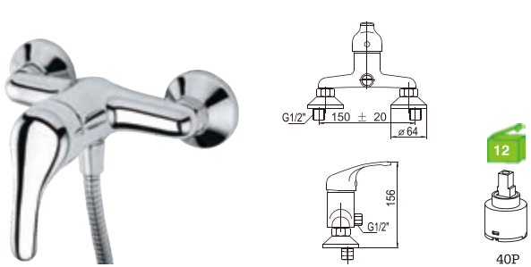
C15DF3C Monocomando duche Shower mixer Monomando ducha C/CHUVEIRO---168 BICHA ---2031(1.7M) SUPORTE ---JH 24.00€ (+IVA)
