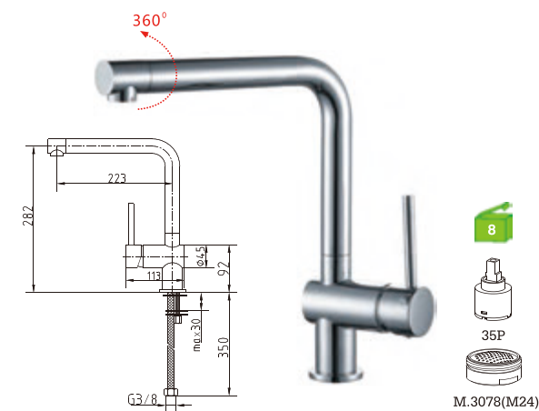
E34FM18C C/bicha certificada Monocomando lava-loiça bica giratório Kitchen mixer swivel spout Monomando fregadero caño giratório 54.00€
