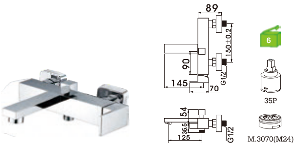
C51FX2C Monocomando banheira Bath/shower mixer Monomando baño C/CHUVEIRO---922 BICHA ---2030CR(1.7M) SUPORTE ---KH INVERSOR ---3036
