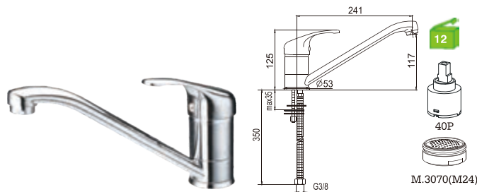
C15DF5C Monocomando lava-loiça Kitchen mixer Monomando fregadero (caño baixo) C/bicha certificada 15.10€ (+IVA)
