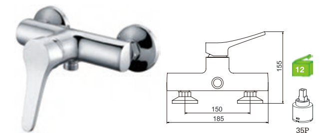
C38DA3C Monocomando duche Shower mixer Monomando ducha C/CHUVEIRO ---168 BICHA ---2031(1.7M) SUPORTE ---JH
