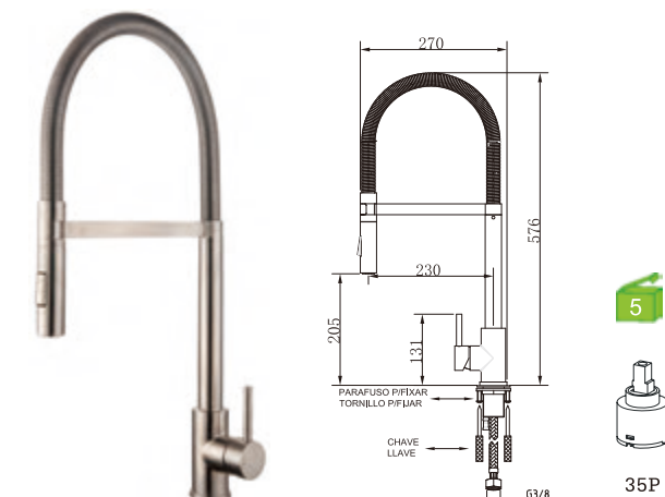
H30LA17X Monocomando de lava-loiça industrial Industry kitchen mixer Monomando de fregadero industrial
