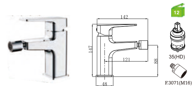
E21BF4C Monocomando bidé Bidet mixer Monomando bidet
