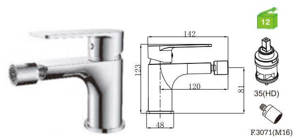
E22BH4C Monocomando bidé Bidet mixer Monomando bidet
