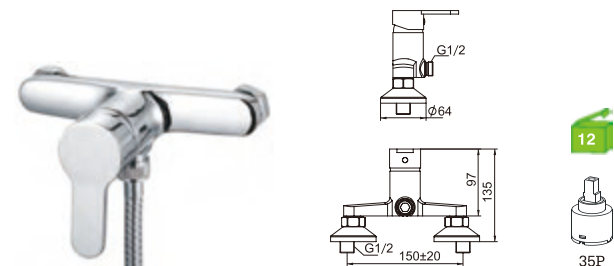
C08GS3C Monocomando duche Shower mixer Monomando ducha C/CHUVEIRO ---168 BICHA ---2031(1.7M) SUPORTE ---JH
