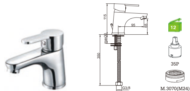
C08GS1C Monocomando lavatório Basin mixer Monomando lavabo
