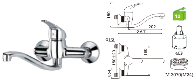
C15DF6C Monocomando lava-loiça à parede bica baixa Wall mounted kitchen mixer Monomando fregadero pared (caño baixo) BICHA ---3060 24.70€ (+IVA)
