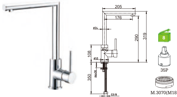
C45GB8C Monocomando lava-loiça Kitchen mixer Monomando fregadero
