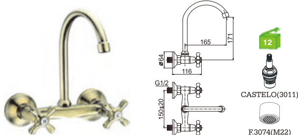
H15T9BR Misturadora lava-loiça à parede bica alta Wall mouted kitchen mixer Monobloc fregadero pared (caño alto) BICA ---3068(BR)
