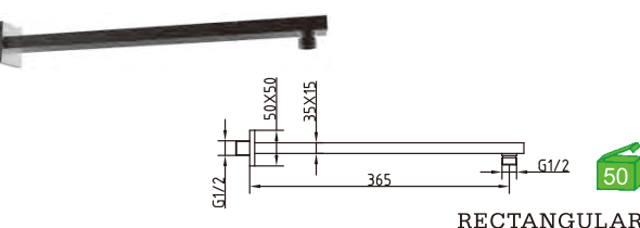
E-D704BL Haste de parede Barra de pared 22.00€ (+IVA)
