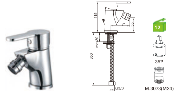
C08GS4C Monocomando bidé Bidet mixer Monomando bidet
