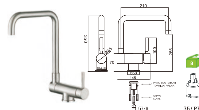
S30LN8X Monocomando de lava-loiça rebatível Kitchen mixer Monomando de fregadero abatible
