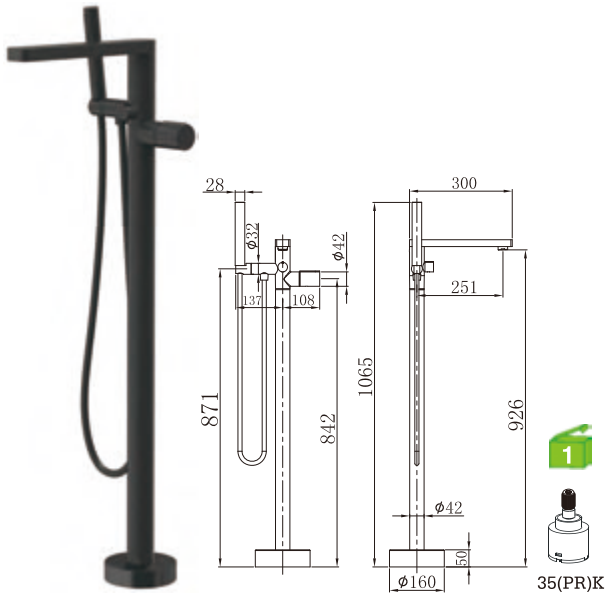
D25WR25BL Monocomando de banheira e duche, montagem ao chão Single-lever bath/shower mixer, floor-mounted Monomando para baño y ducha de pie 269.00€ (+IVA)
