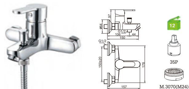
C08GS2C Monocomando banheira Bath/shower mixer Monomando baño C/CHUVEIRO ---168 BICHA ---2031(1.7M) SUPORTE ---JH
