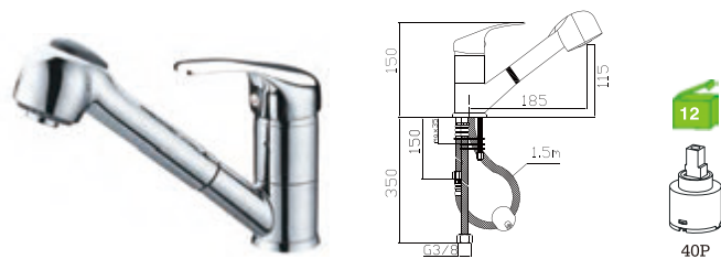
C15DF7C Monocomando lava-loiça com chuveiro Kitchen mixer with pull out shower Monomando fregadero extraíble C/CHUVEIRO---172 BICHA ---2028(1.5M) 24.80€ (+IVA)
