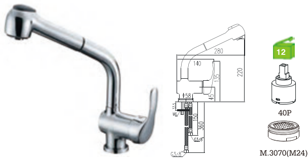
C17DF7C Monocomando lava-loiça com chuveiro Kitchen mixer with pull out shower Monomando fregadero extraíble C/CHUVEIRO---172 BICHA ---2028(1.5M) 31.30€ (+IVA)
