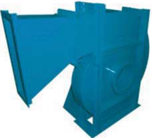
BCN 后弯高压风机 叶轮直径：27 至73 in. (685 至1,854 mm) 风量：至75,000 CFM (127,425 m 3 /h) 静压：至100 in. w.g. (24,863 Pa) 样本号：1450
