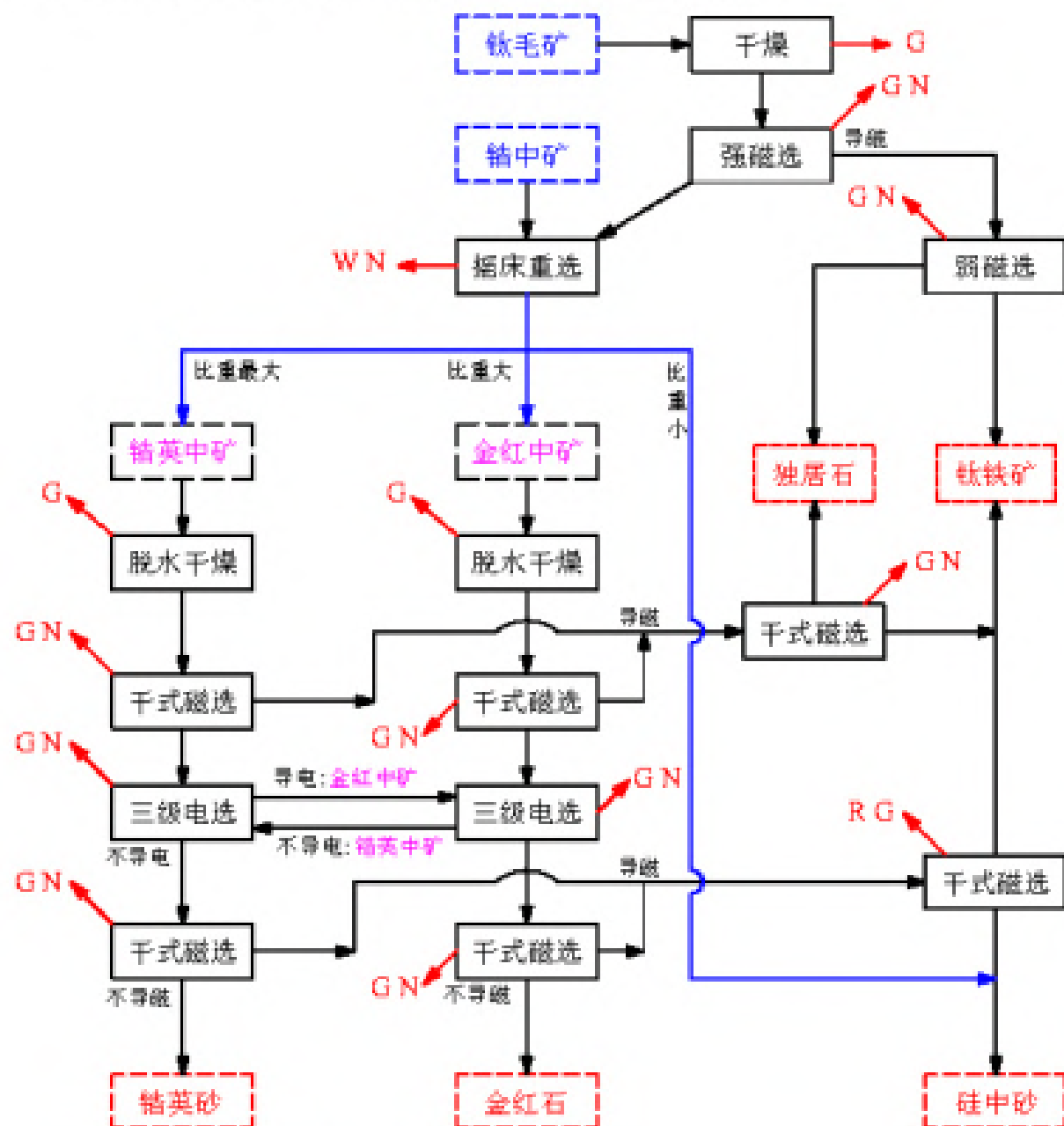
图 3.6-1 钛毛矿及锆中矿选矿工艺主要产污环节图
