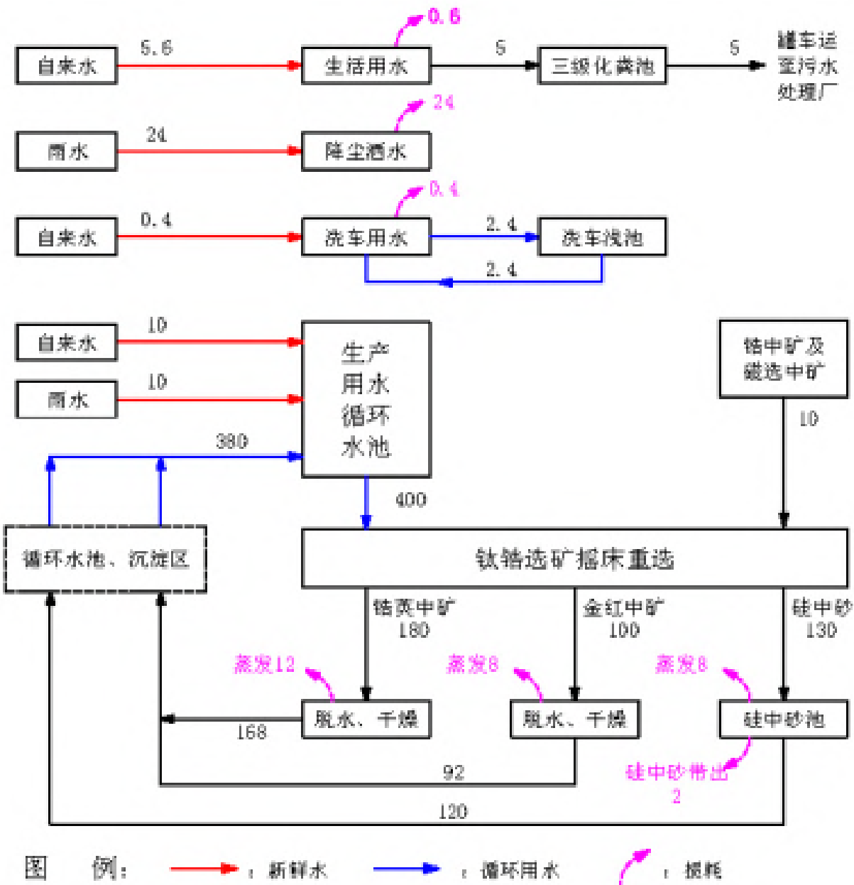
图 3.5-5 项目非雨季水平衡图 (单位: m³/d)
