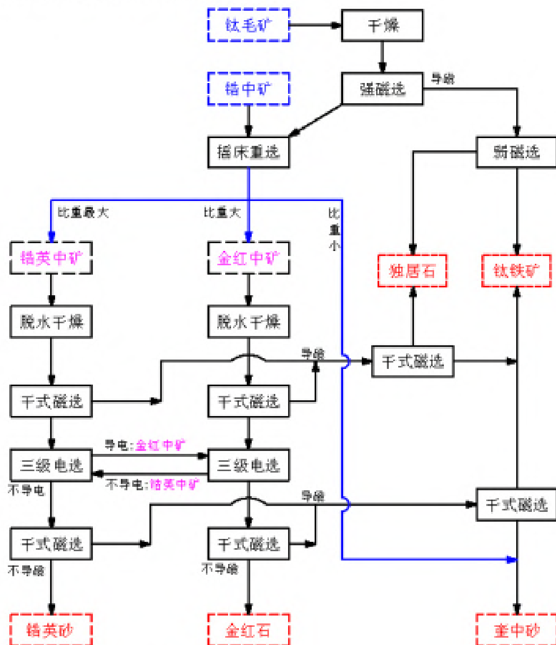
图 3.5-1 钛铁矿及锆中矿选矿工艺流程
