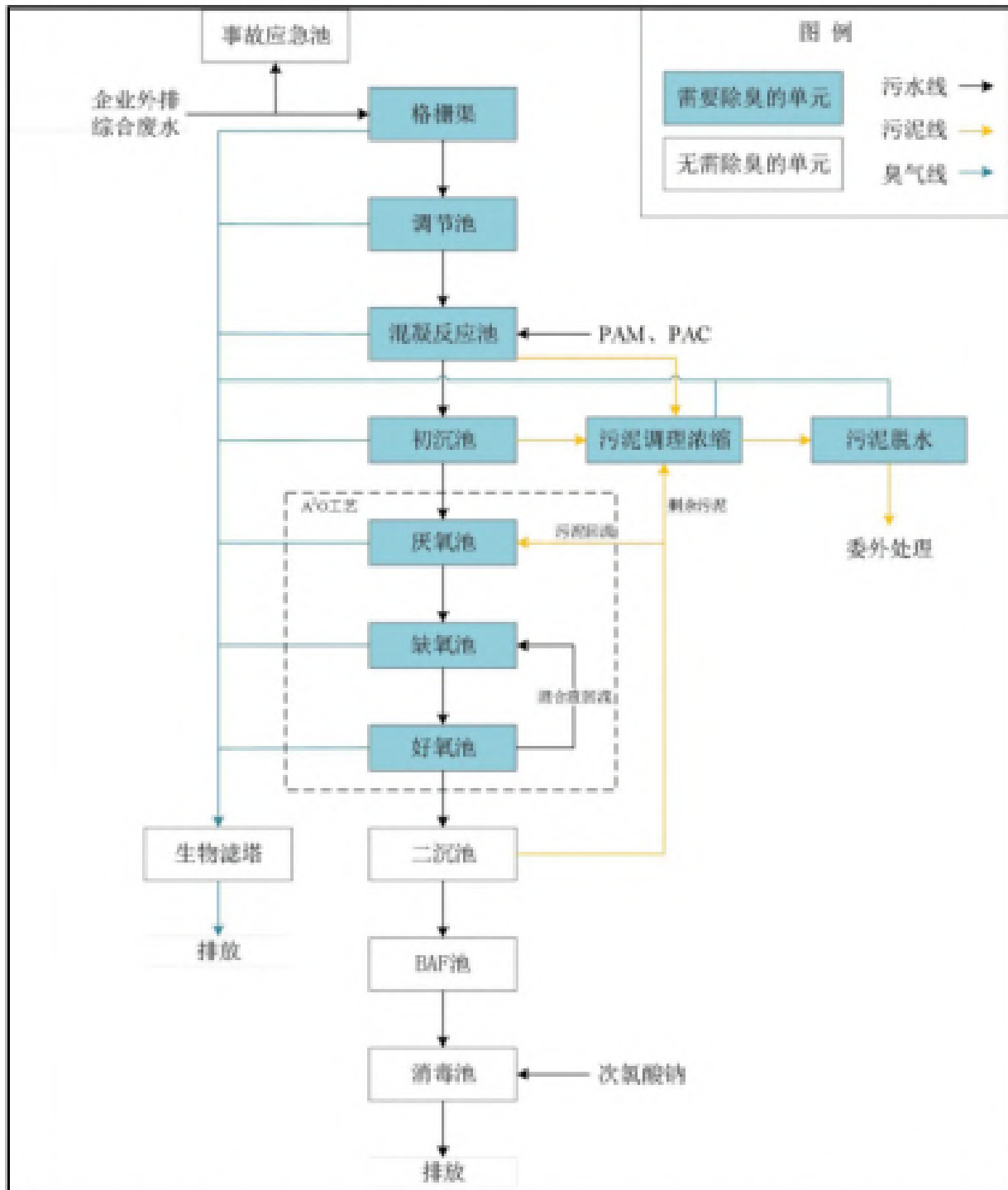
图 6.2-4 阳西县新墟产业园污水处理厂（一期）污水处理工艺流程图
