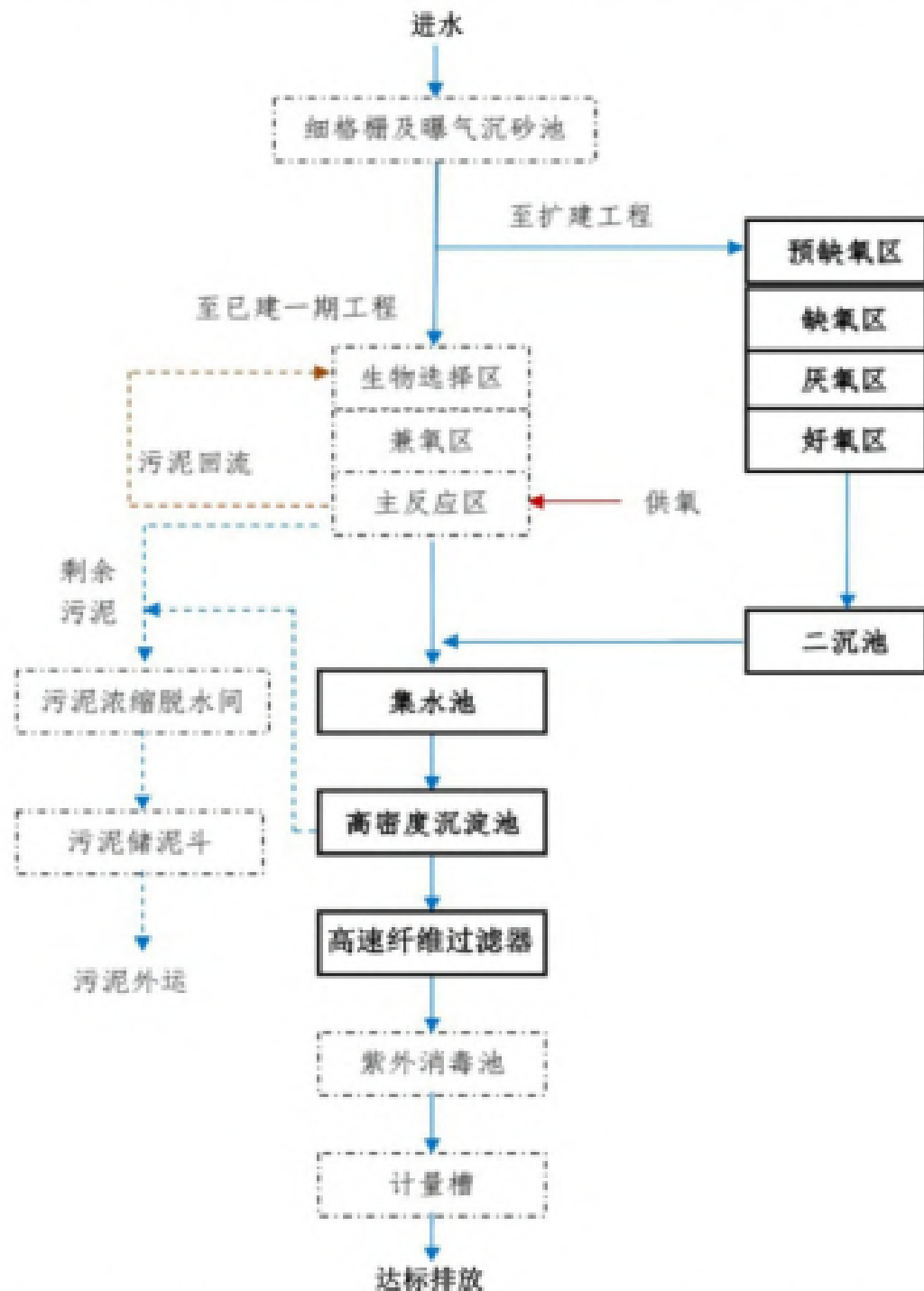
图 6.2-3 中山火炬（阳西）产业转移工业园污水处理厂污水处理工艺流程
