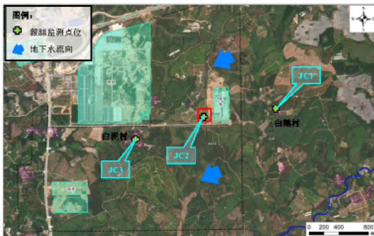
图 6.3-2 地下水环境跟踪监测点位布置示意图
