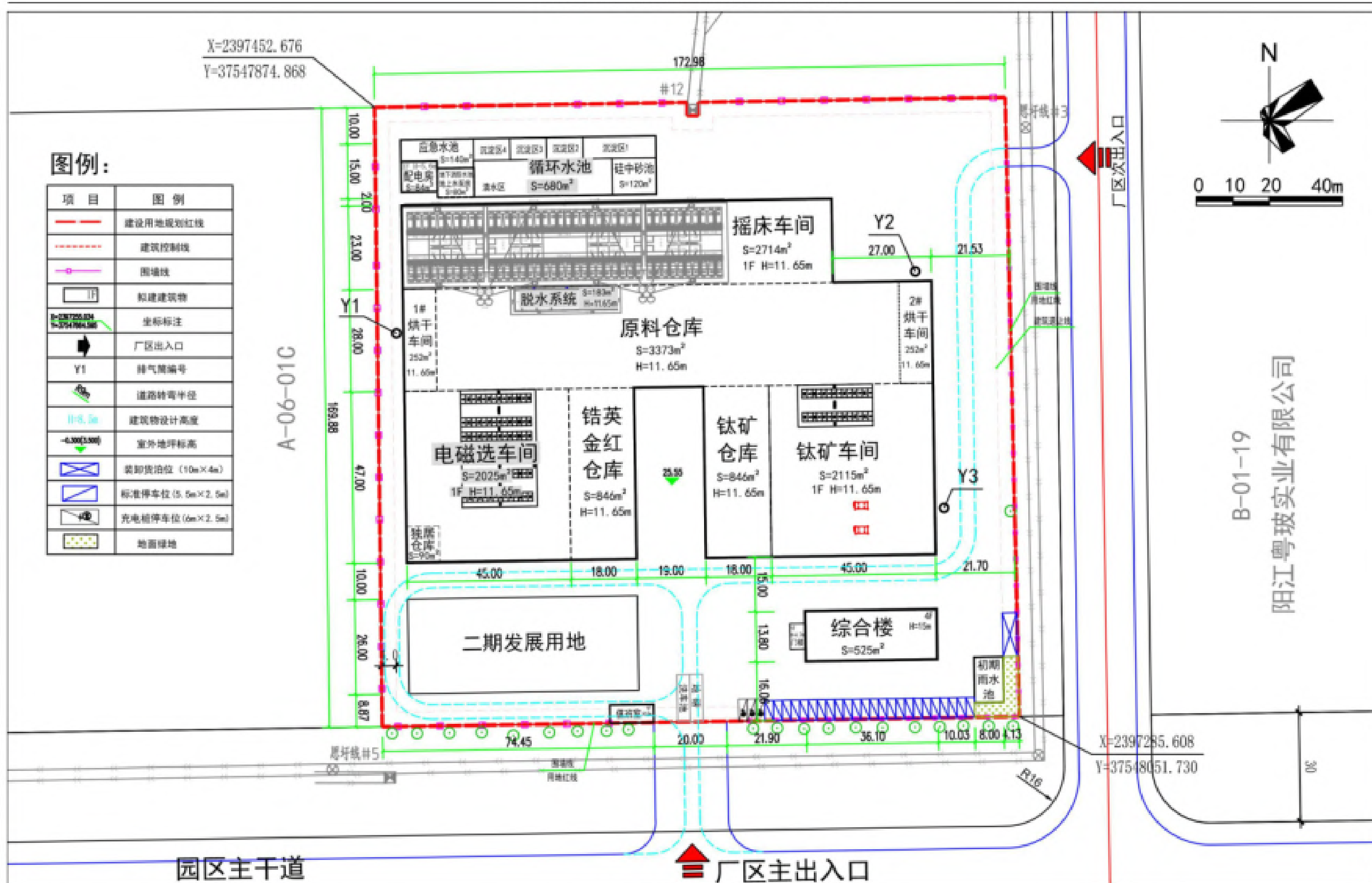
图 3.3-1 本项目厂区总平面布置图
