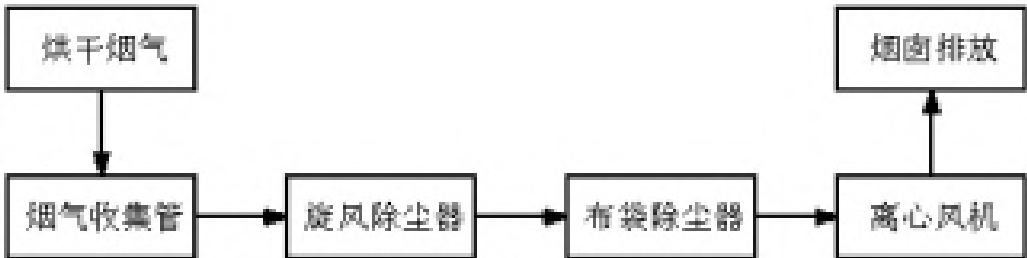
图6.4-1 “旋风+布袋除尘”措施工艺流程图
