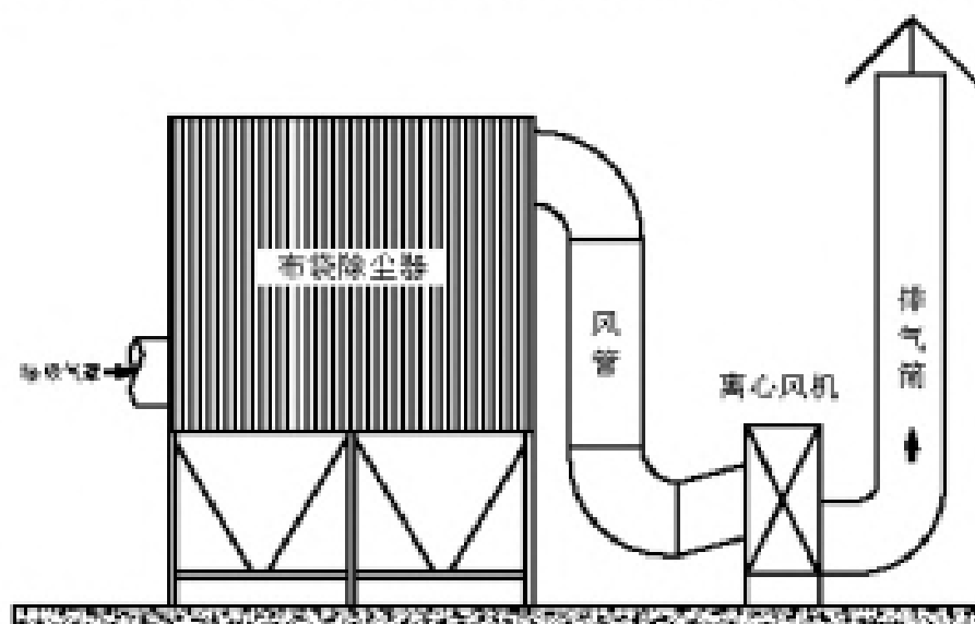
图 6.4-3 干选工序布袋除尘系统示意图
