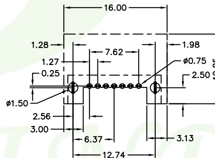
P.B.C Layout
