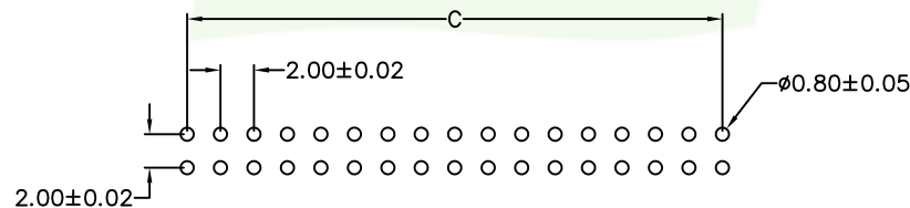
P.C.Board Layout
