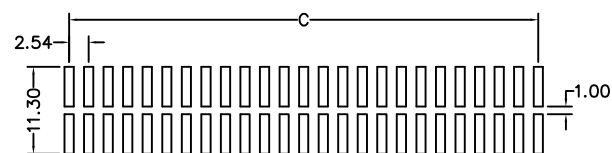
P.C.Board Layout
