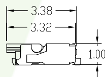
SECTION A-A 3:1
