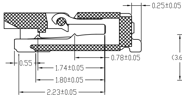
SECTION A-A 3:1
