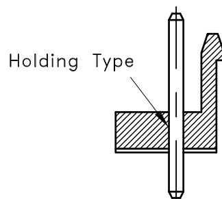
A-A SEC
