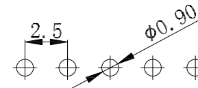
P.C.B Hole Layout
