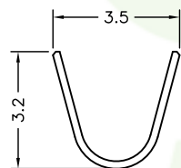
A-A SEC
